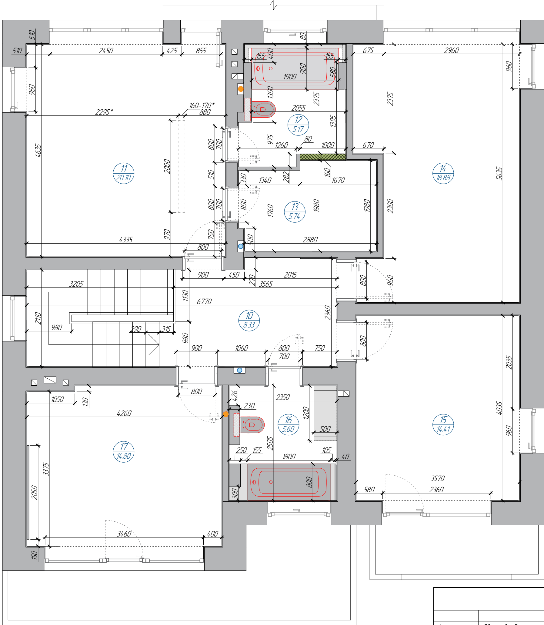
План 2 этажа
