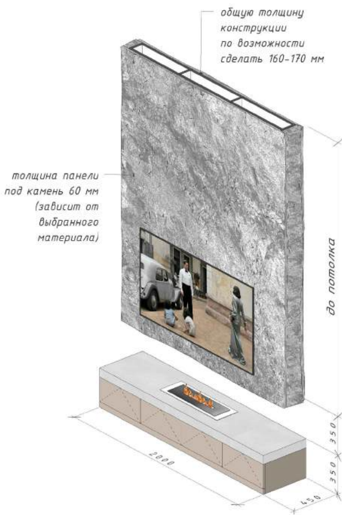
Схема подвесной конструкции под ТВ в спальне
