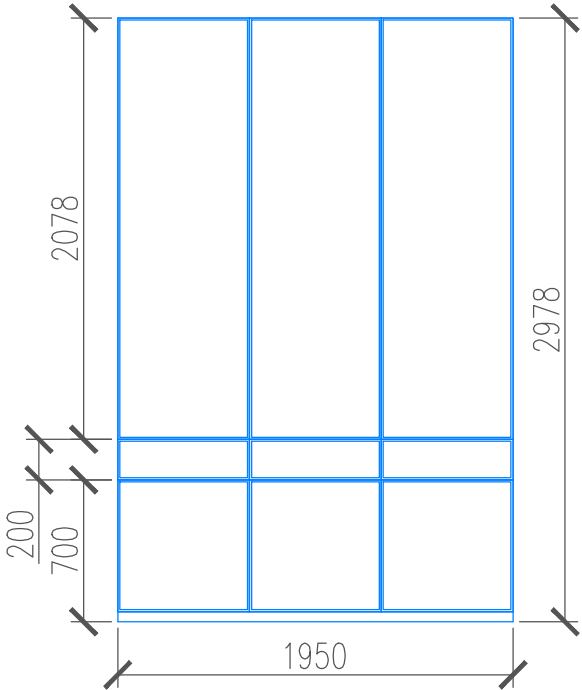
Глубина шкафа –600мм
