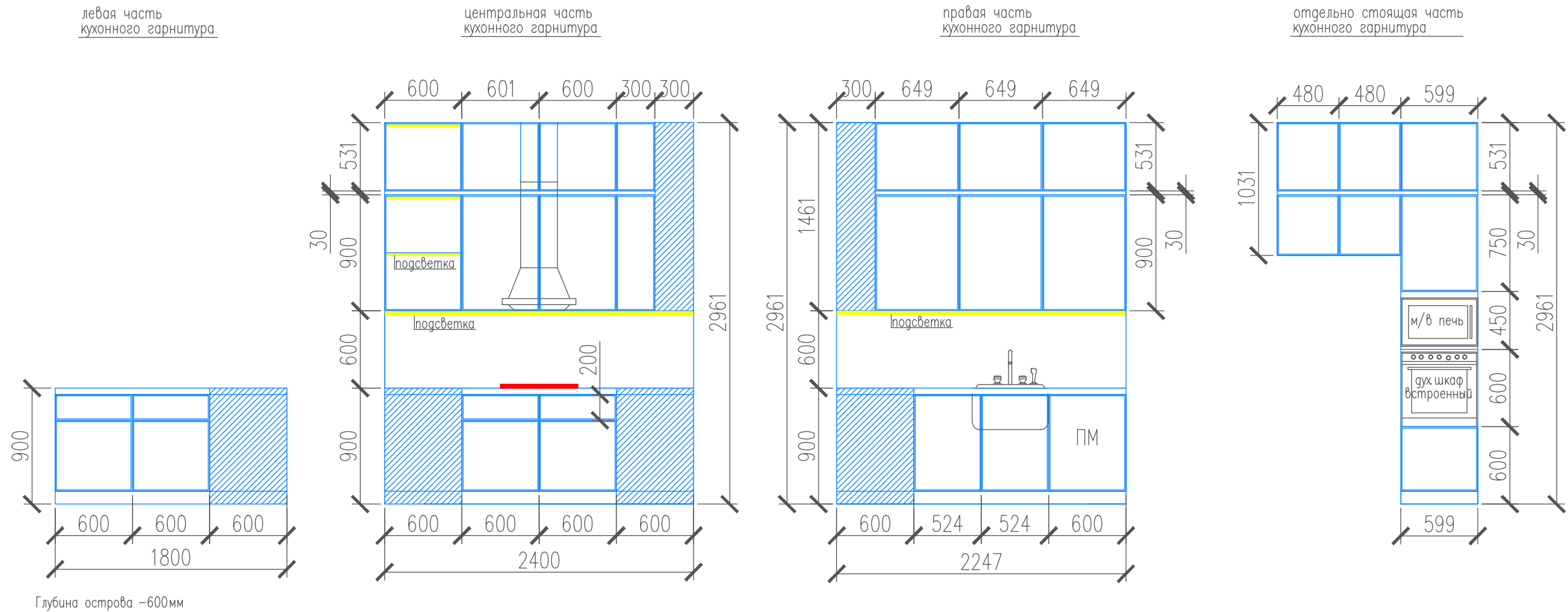
Кухонный гарнитур
