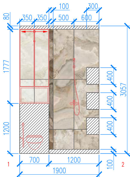
Развертка короба инсталляции
