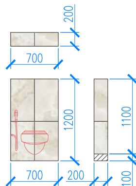
Развертка короба инсталляции
