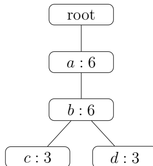
Hình 3: FP-tree cho CSDL Bảng 8. Node b phân nhánh thành c và d nên cây không phải single-path.
