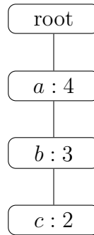
Hình 4: FP-tree cho CSDL Bảng 10. Không node nào phân nhánh nên cây là single-path, FP-Max trả thẳng một tối đại.
