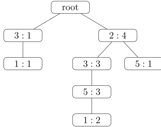
Hình 2: FP-tree cho CSDL toy Bảng 5 sau bước tĩa và sắp thứ tự (Bảng 6).
