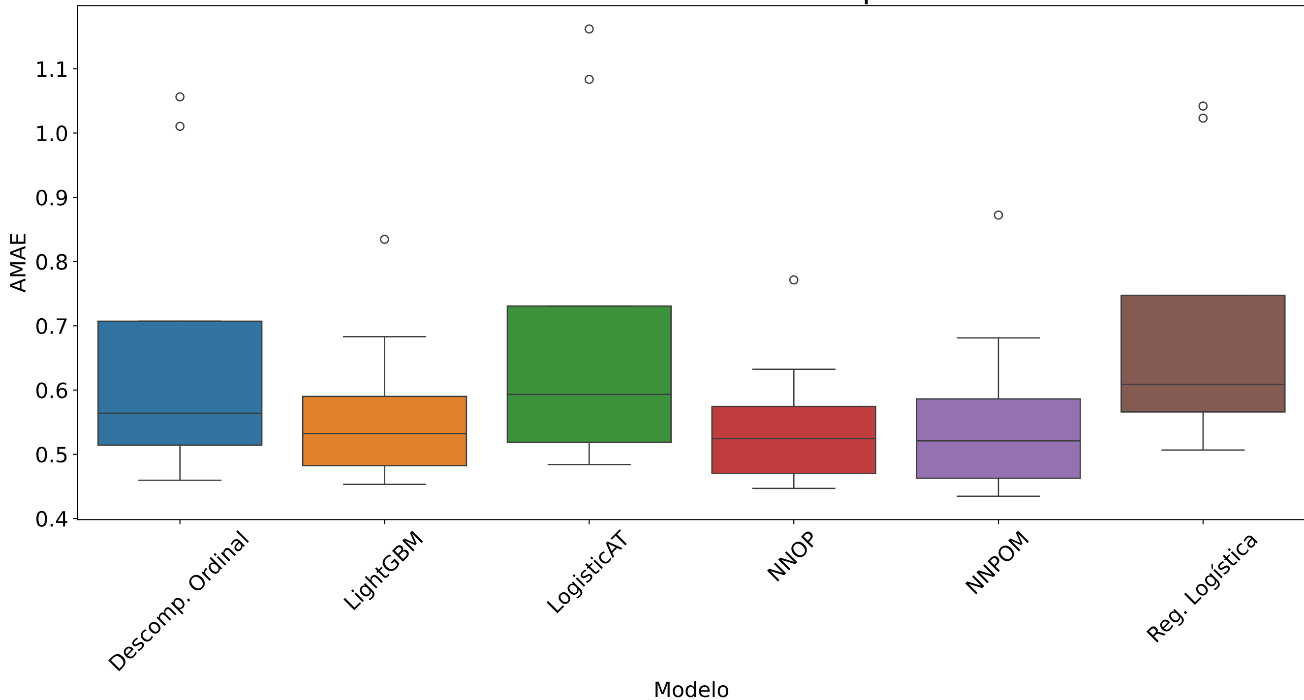
Distribución de la métrica AMAE por Modelo
