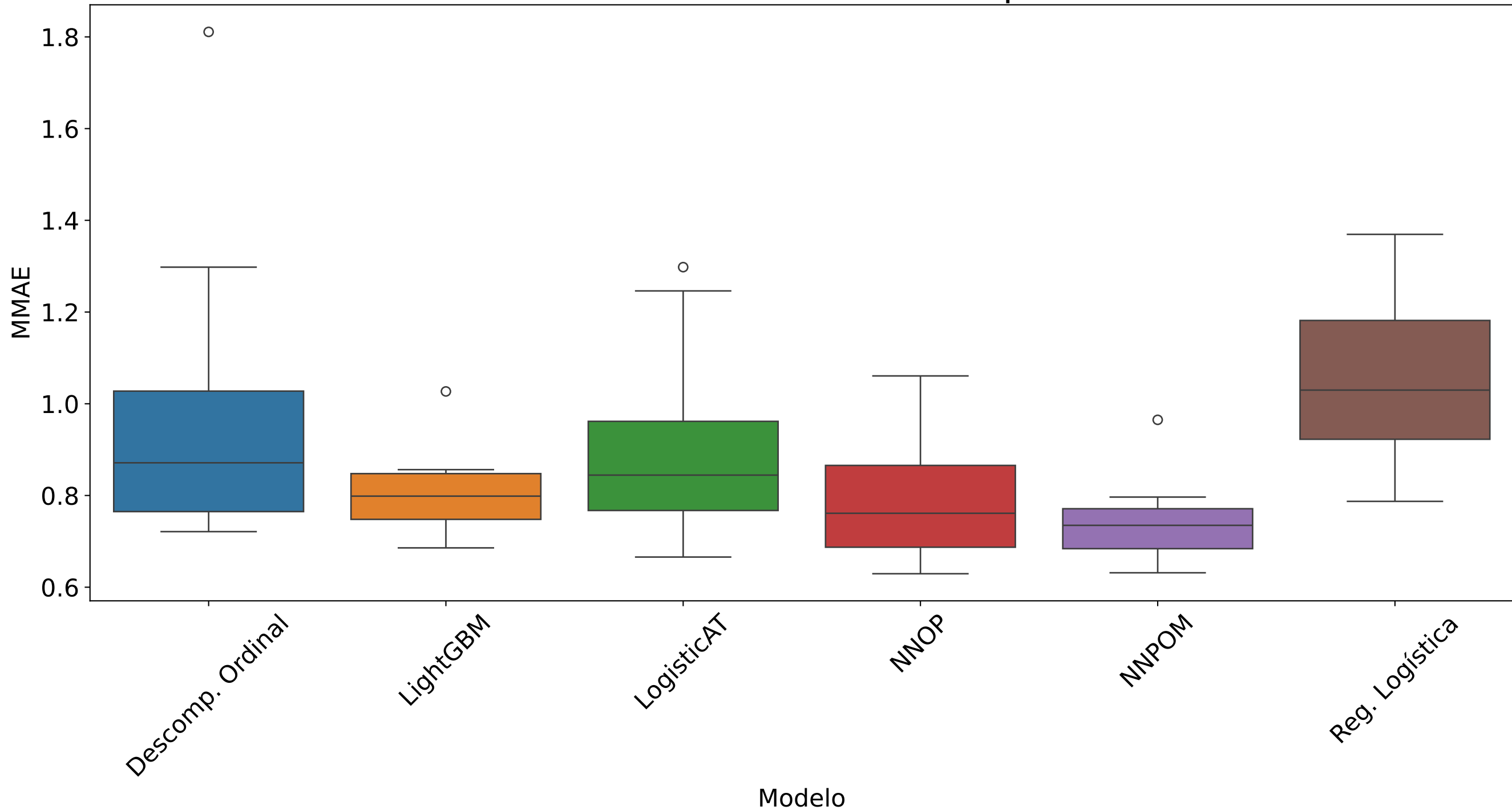
Distribución de la métrica MMAE por Modelo
