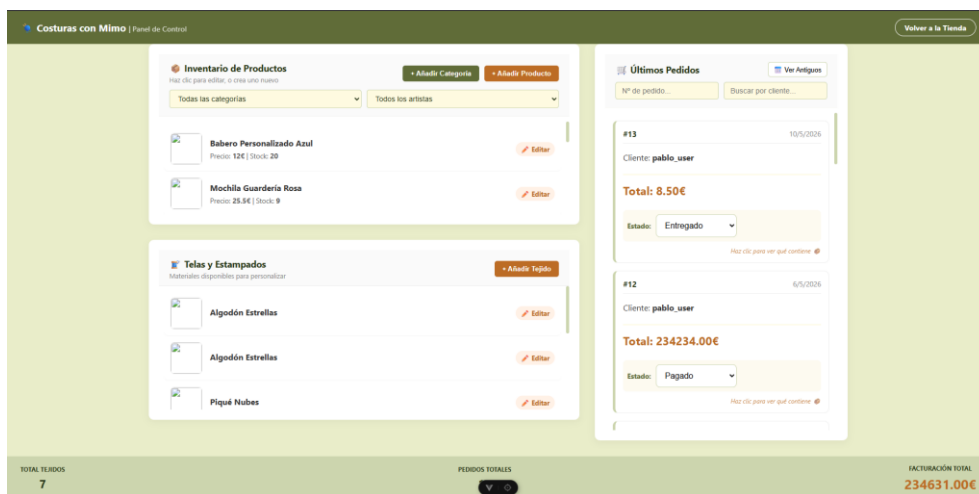
Ilustración 14 Dashboard
