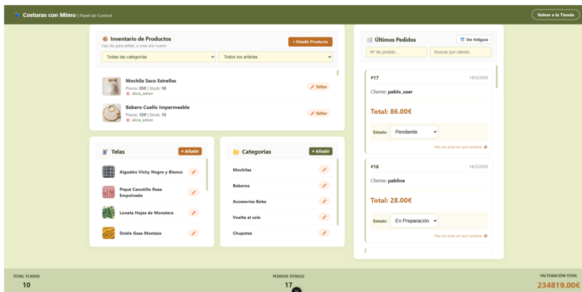
Ilustración 14 Dashboard
