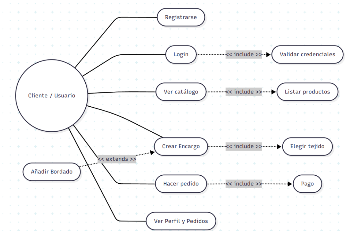
Ilustración 2 Caso de uso Cliente
