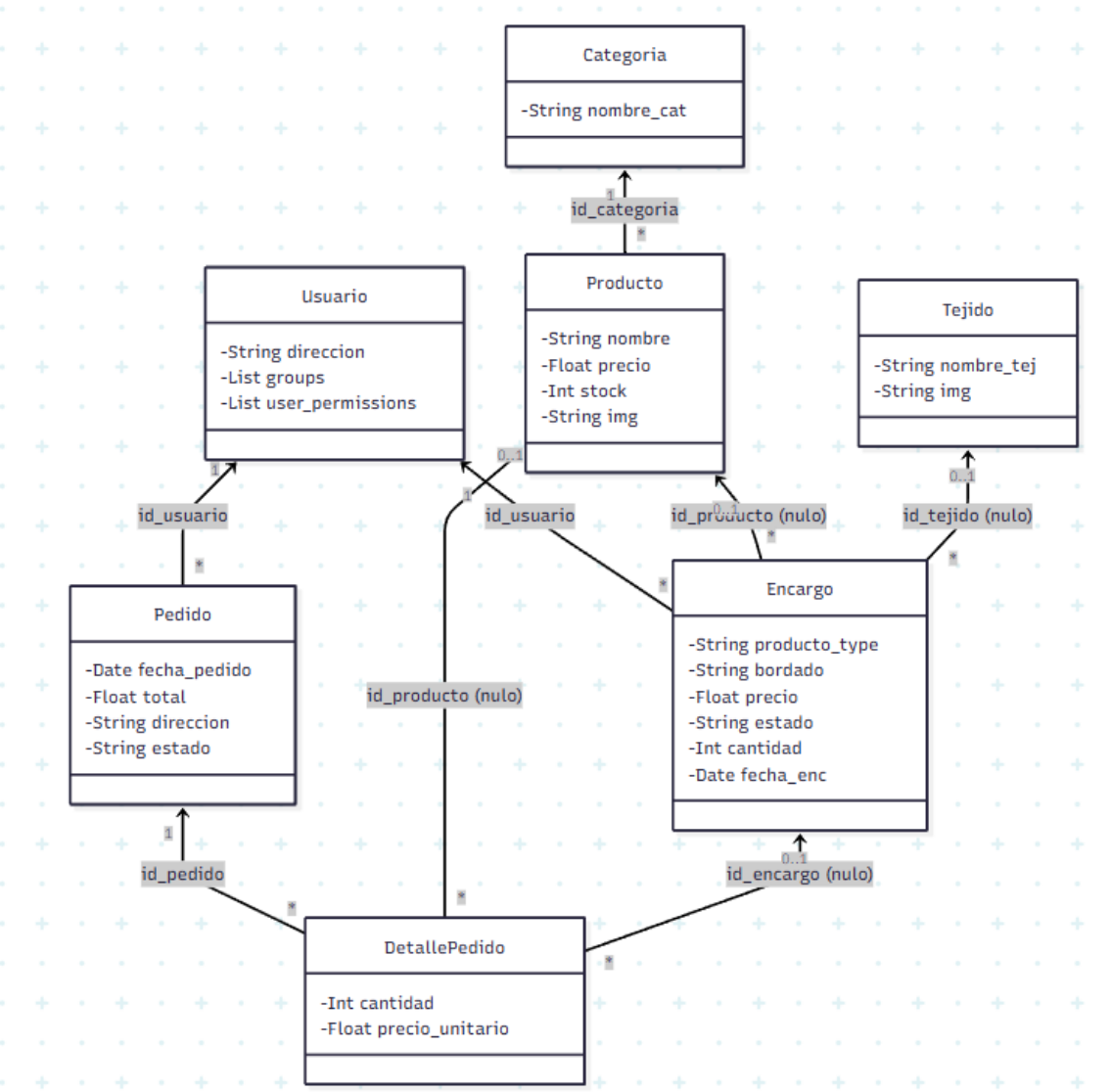
Ilustración 4 Diagrama de Clases
