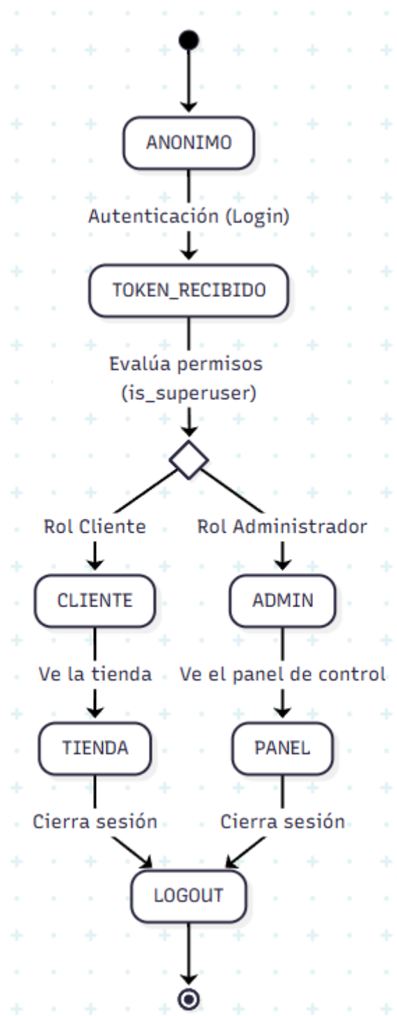
Ilustración 6 Diagrama de estados Login
