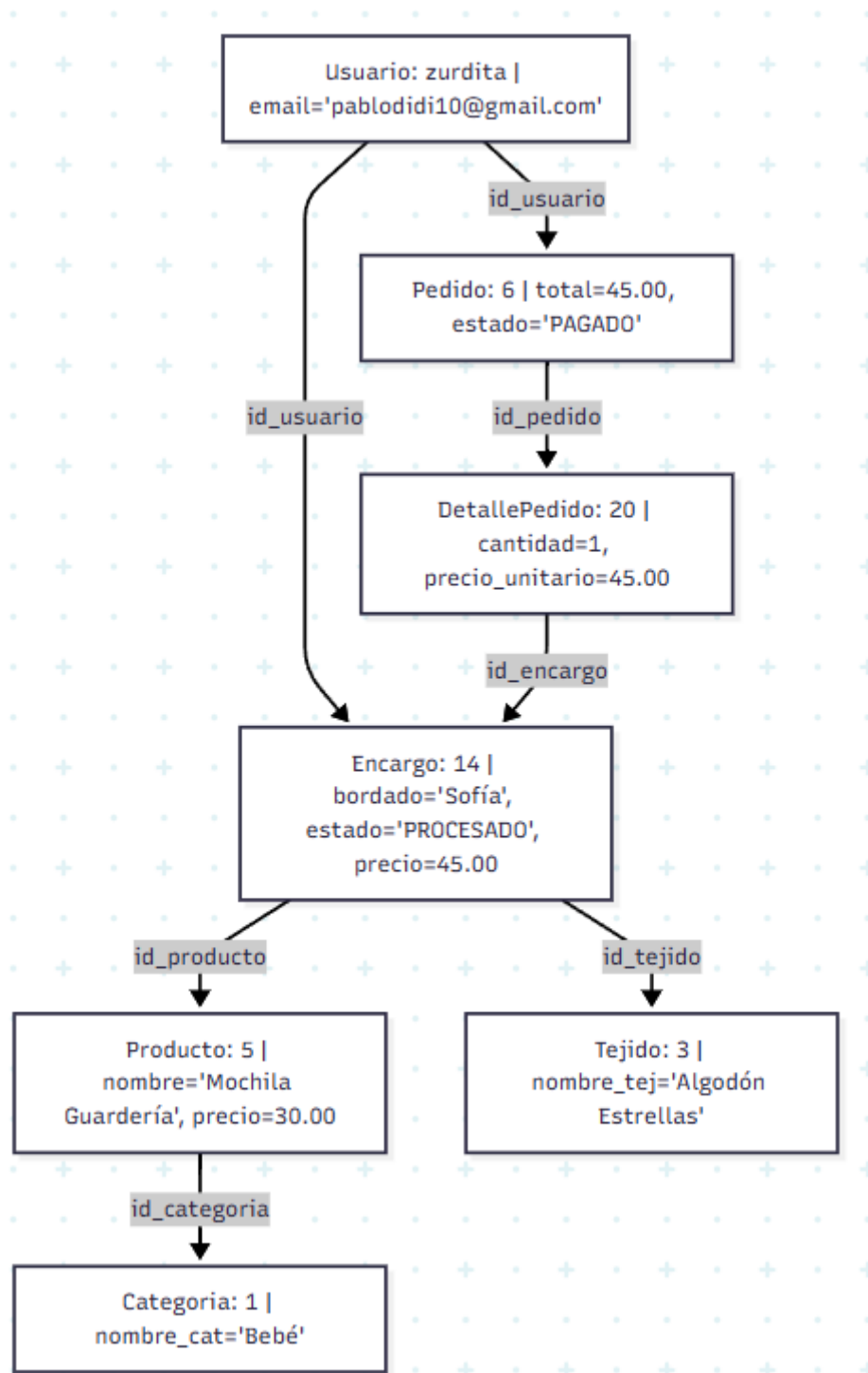
Ilustración 9 Diagrama de objetos
