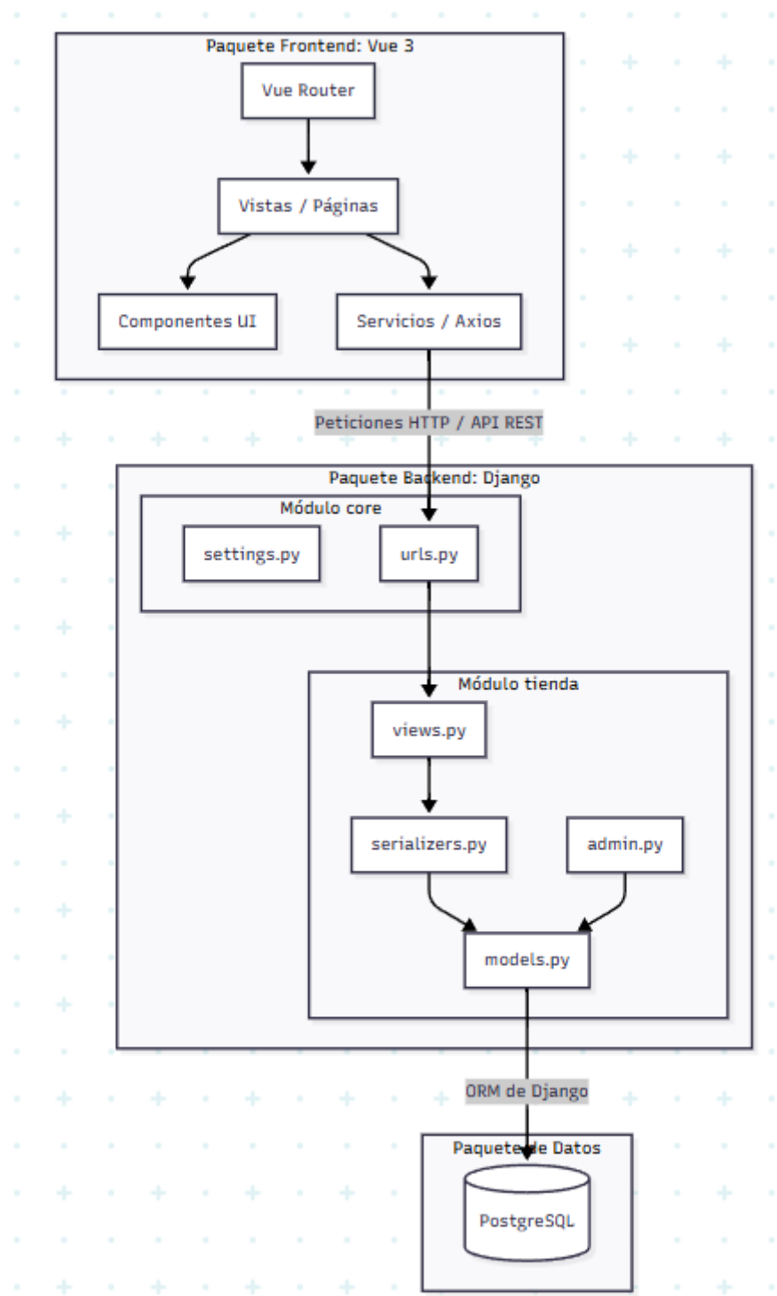
Ilustración 8 Diagrama de paquetes
