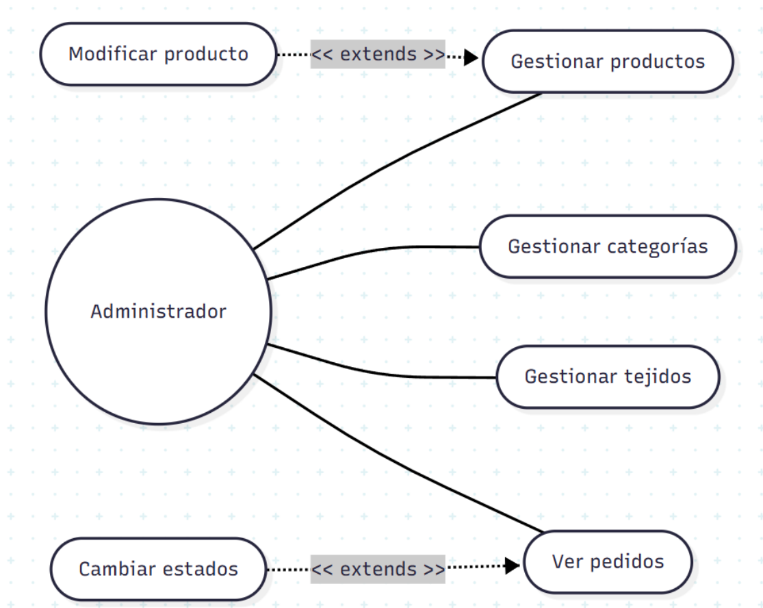
Ilustración 3 Caso de uso Admin
