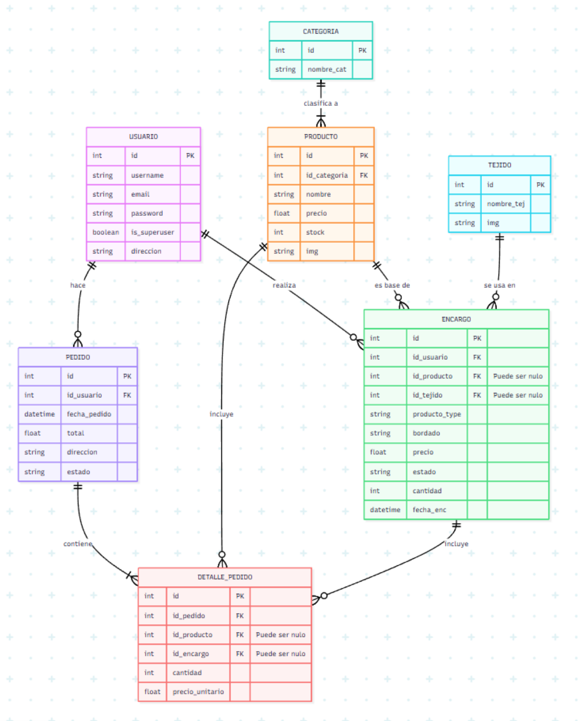
Ilustración 1 Diagrama E/R
