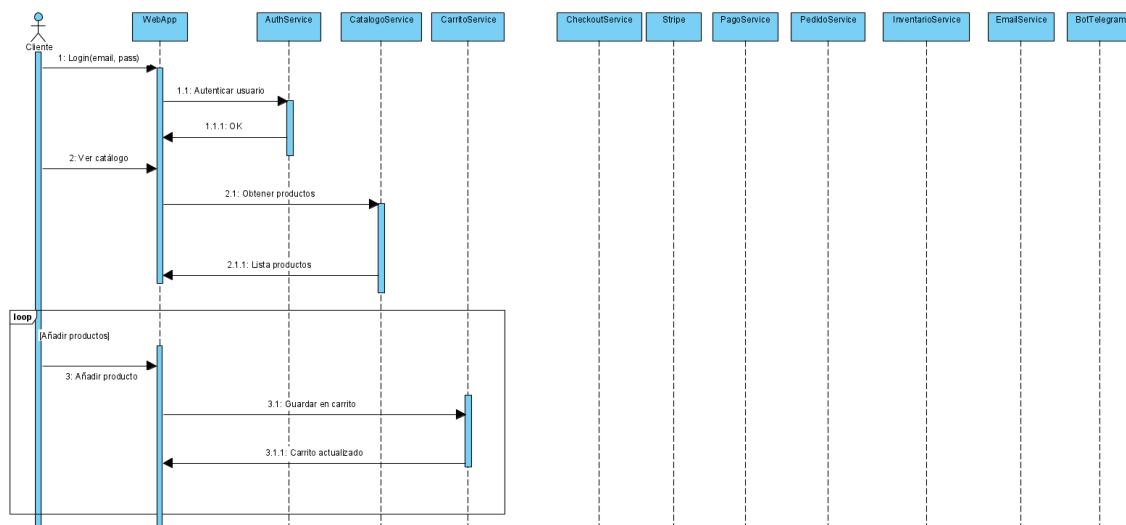
Figura 5.3: Diagrama de secuencia — parte 1: autenticación y carrito
