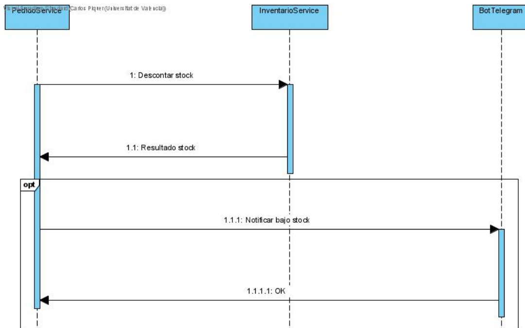
Figura 5.8: Diagrama de secuencia — notificación de bajo stock
