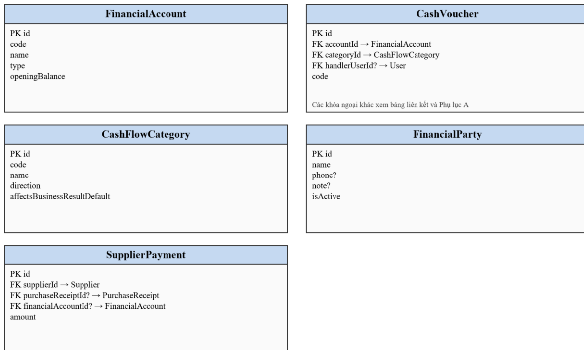
Hình 3.20: Lược đồ quan hệ chi tiết sổ quỹ
