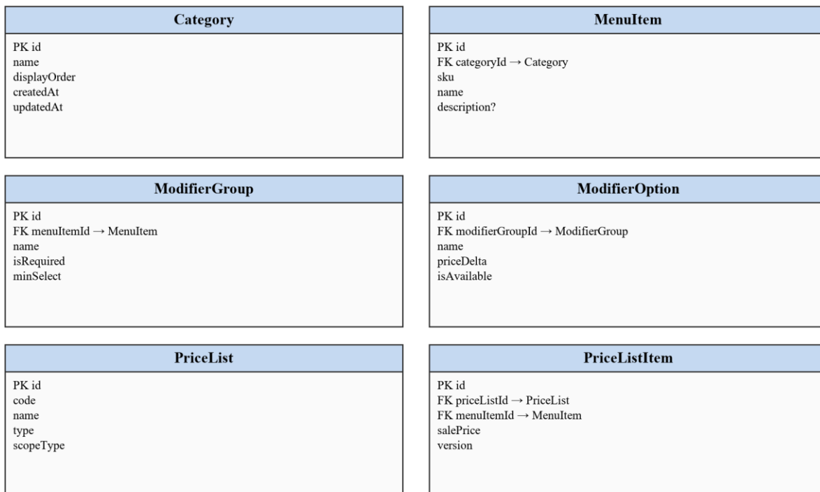
Hình 3.16: Lược đồ quan hệ chi tiết thực đơn và bảng giá
