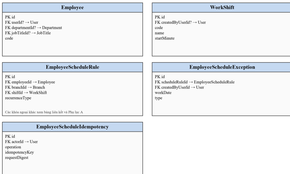
Hình 3.11: Lược đồ quan hệ chi tiết ca làm việc
