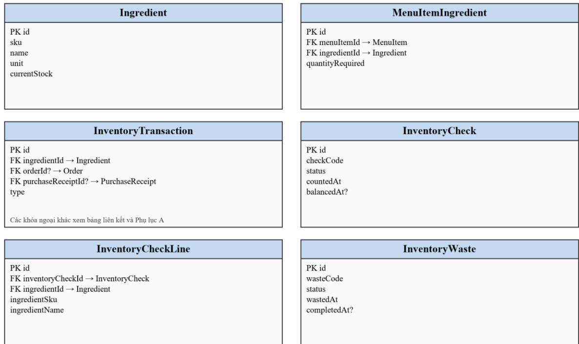
Hình 3.18: Lược đồ quan hệ chi tiết nguyên liệu và định lượng
