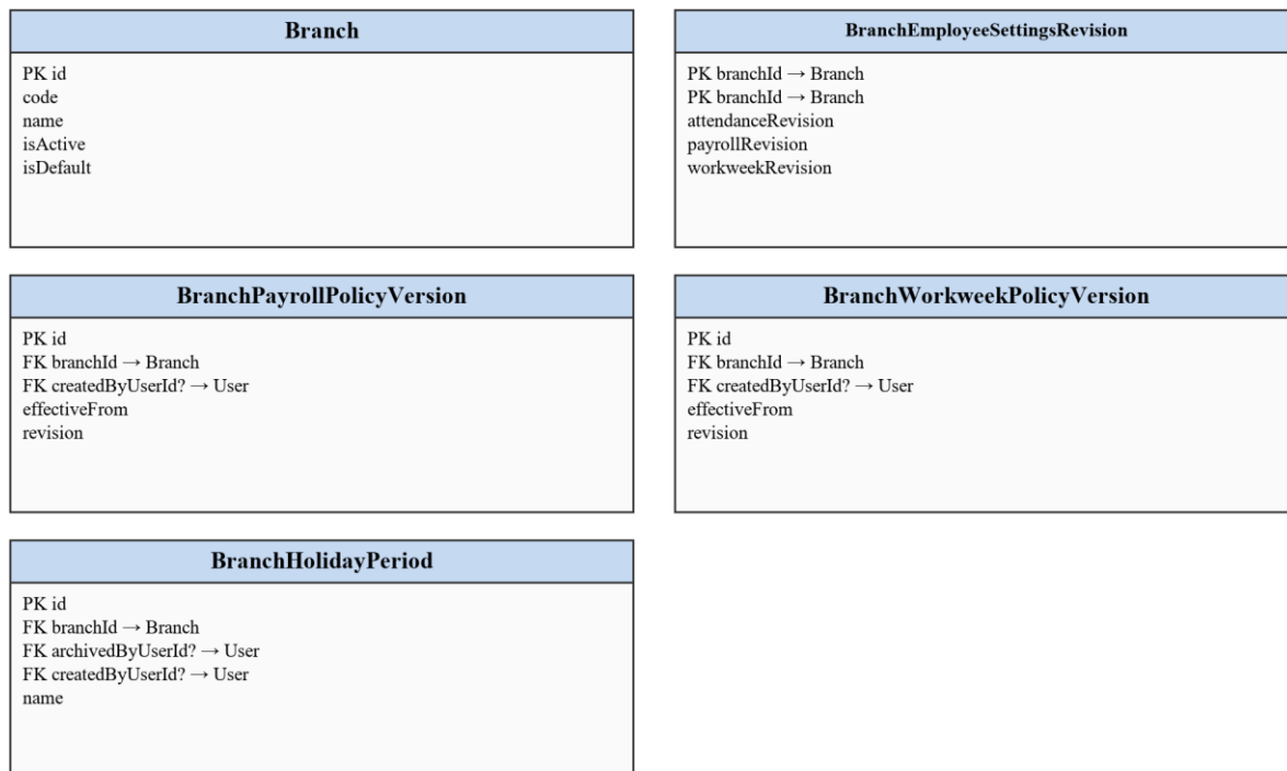
Hình 3.22: Lược đồ quan hệ chi tiết chính sách nhân sự
