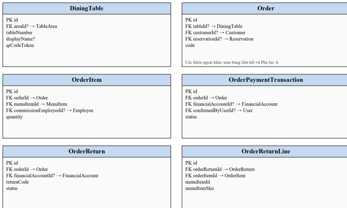
Hình 3.17: Lược đồ quan hệ chi tiết đơn hàng và thanh toán
