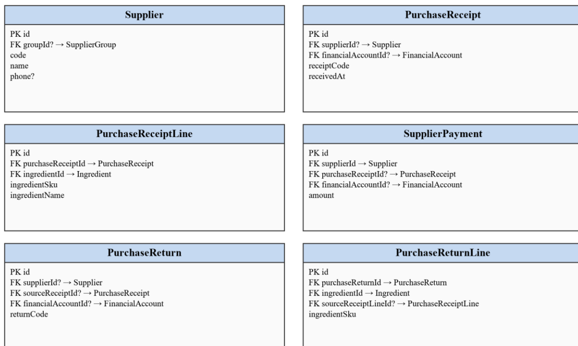
Hình 3.19: Lược đồ quan hệ chi tiết nhập hàng và công nợ
