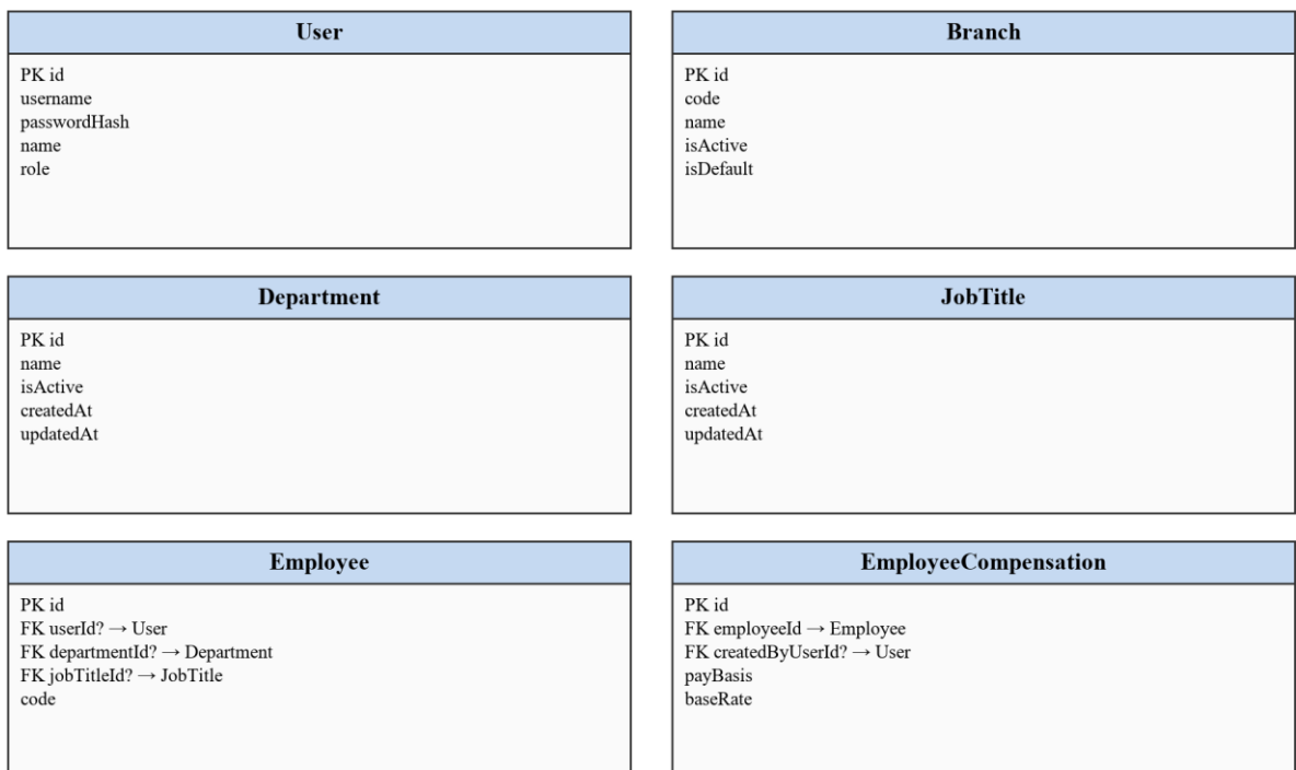
Hình 3.10: Lược đồ quan hệ chi tiết tài khoản, chi nhánh và hồ sơ
