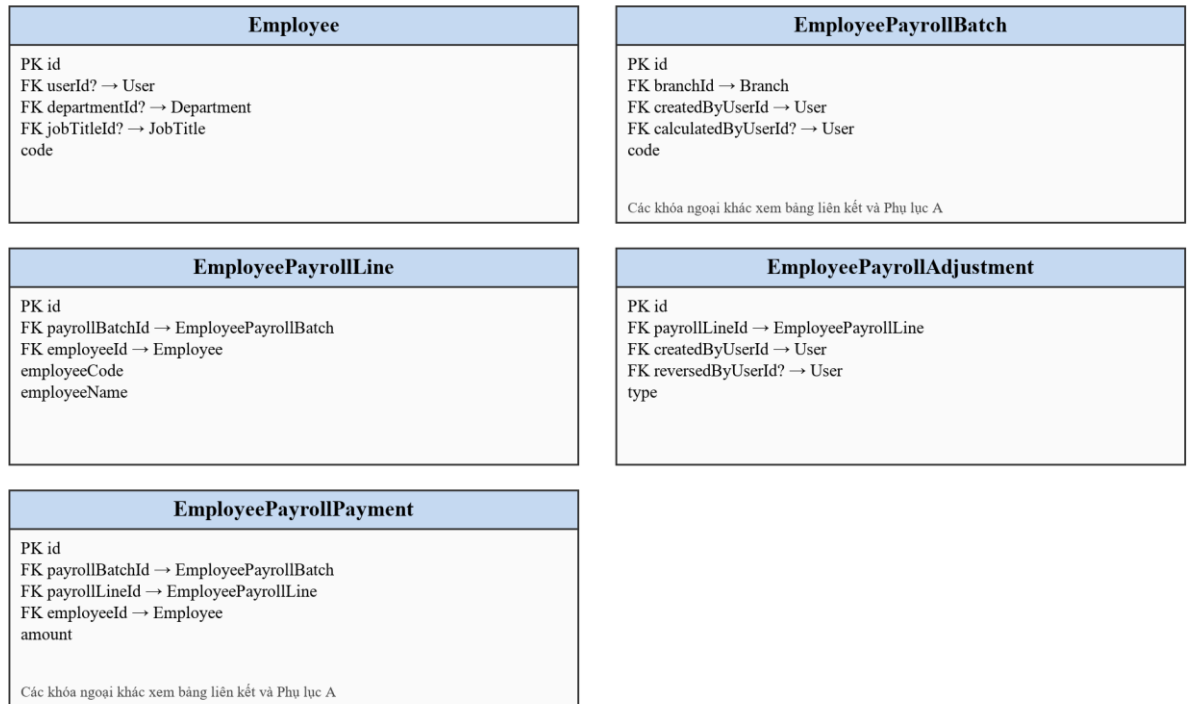
Hình 3.13: Lược đồ quan hệ chi tiết bảng lương
