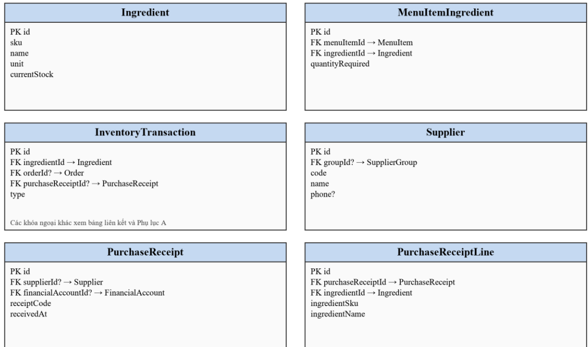
Hình 3.7: Quan hệ dữ liệu kho và mua hàng
