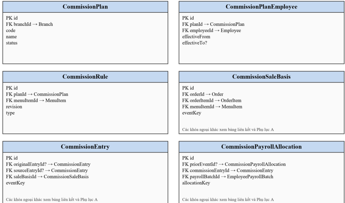
Hình 3.14: Lược đồ quan hệ chi tiết hoa hồng
