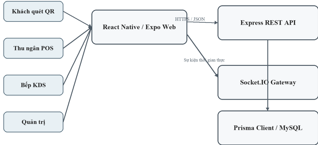
Hình 3.5: Kiến trúc tổng thể hệ thống Crispy Bite
