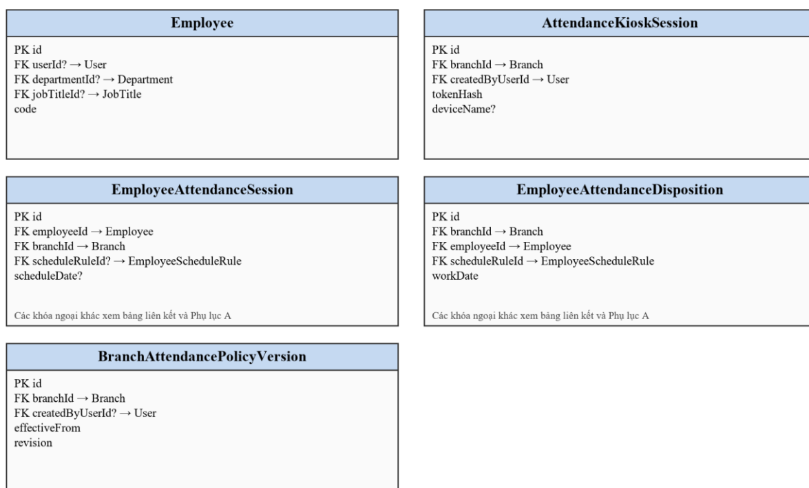
Hình 3.12: Lược đồ quan hệ chi tiết chấm công
