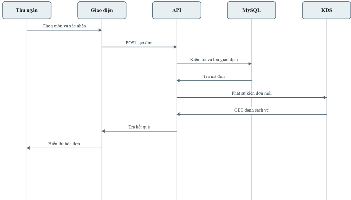
Hình 3.10: Biểu đồ tuần tự tạo đơn và chuyển bếp
