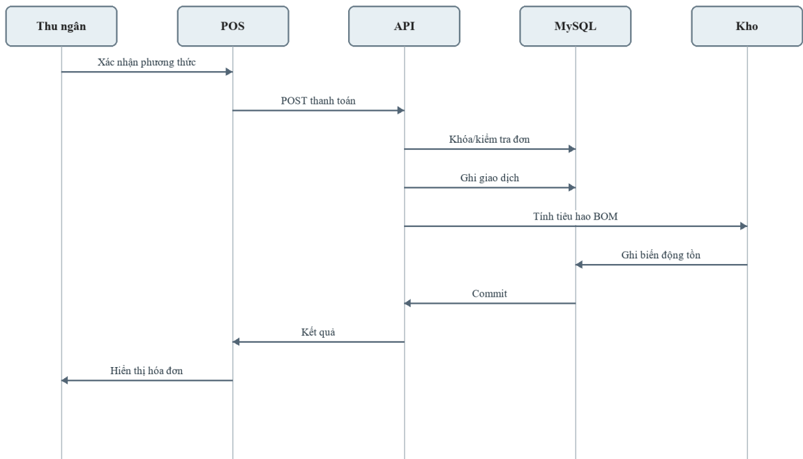
Hình 3.11: Biểu đồ tuần tự thanh toán
