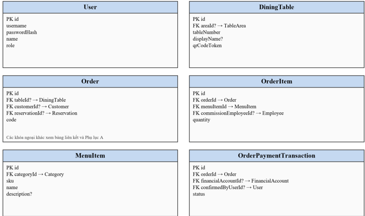
Hình 3.6: Quan hệ dữ liệu đơn hàng
