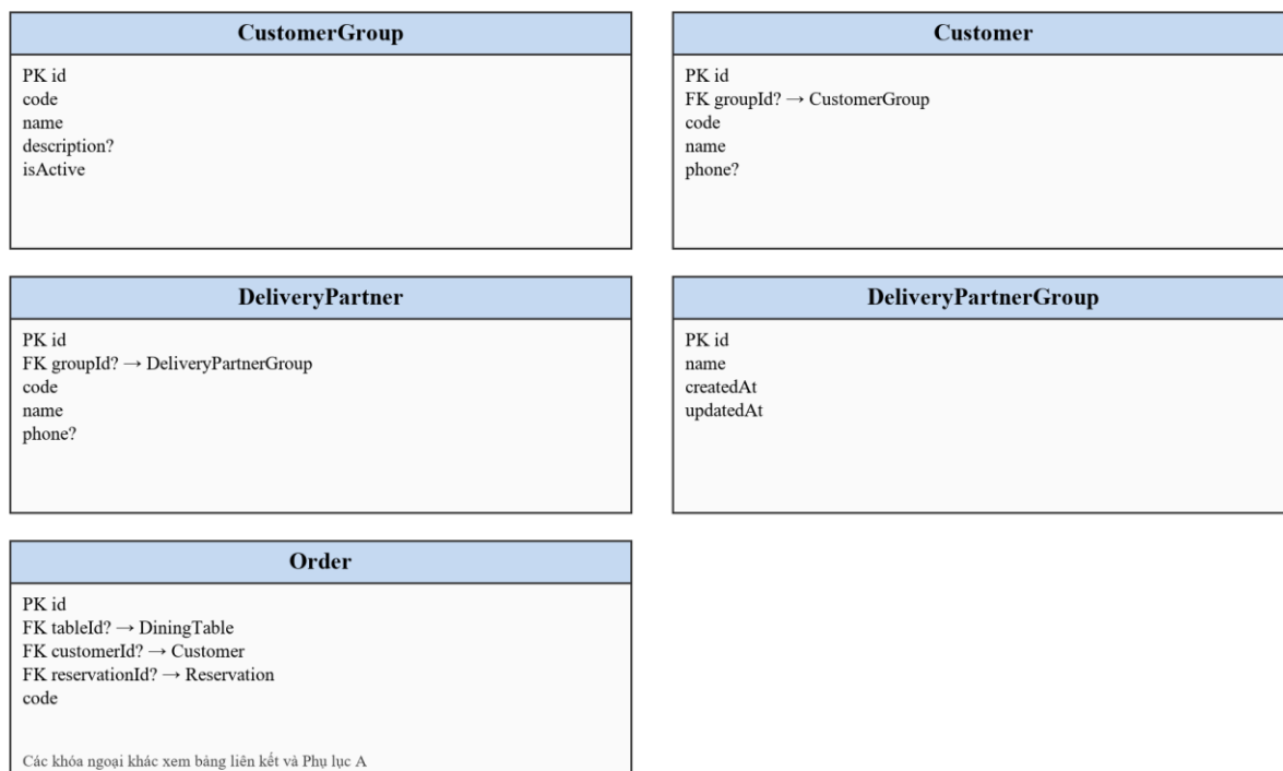
Hình 3.21: Lược đồ quan hệ chi tiết đối tác giao hàng
