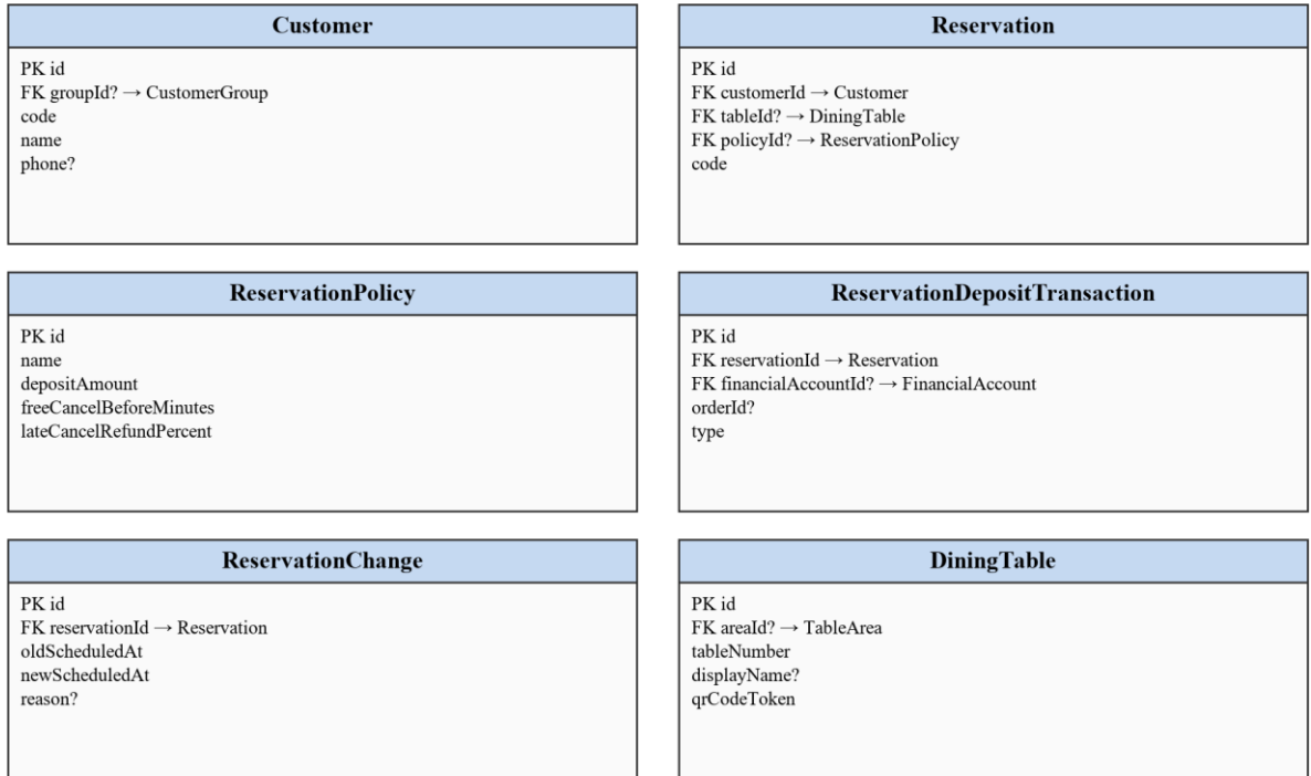
Hình 3.15: Lược đồ quan hệ chi tiết khách hàng và đặt bàn
