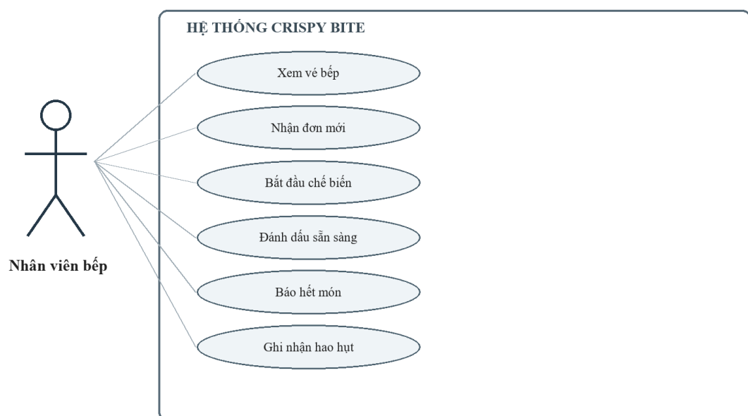
Hình 3.2: Use case bếp
