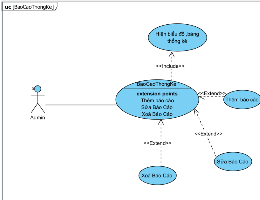
Hình 3. 3: Biểu đồ use-case BaoCao- ThongKe
