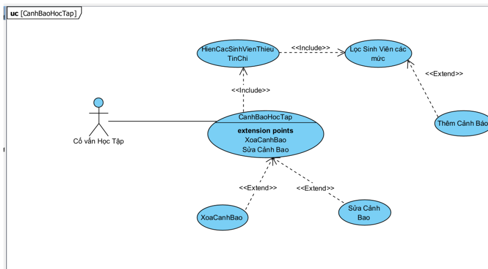
Hình 3. 5: Biểu đồ use-case CanhBaoHocTap
