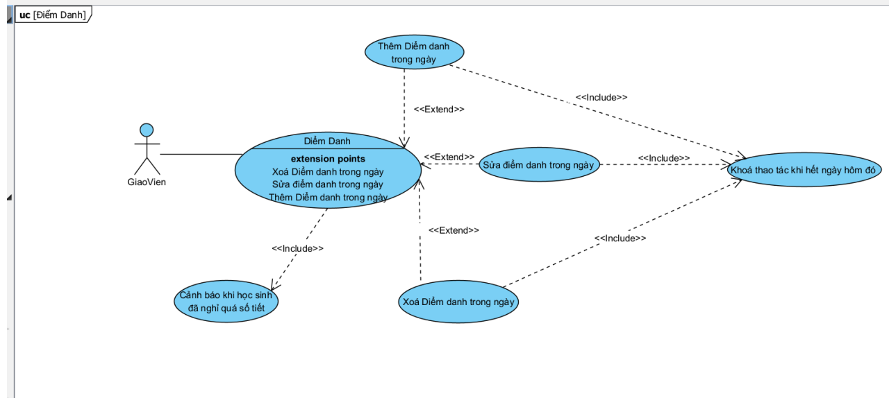
Hình 3. 7: Biểu đồ use-case QuanLyDiemDanh
