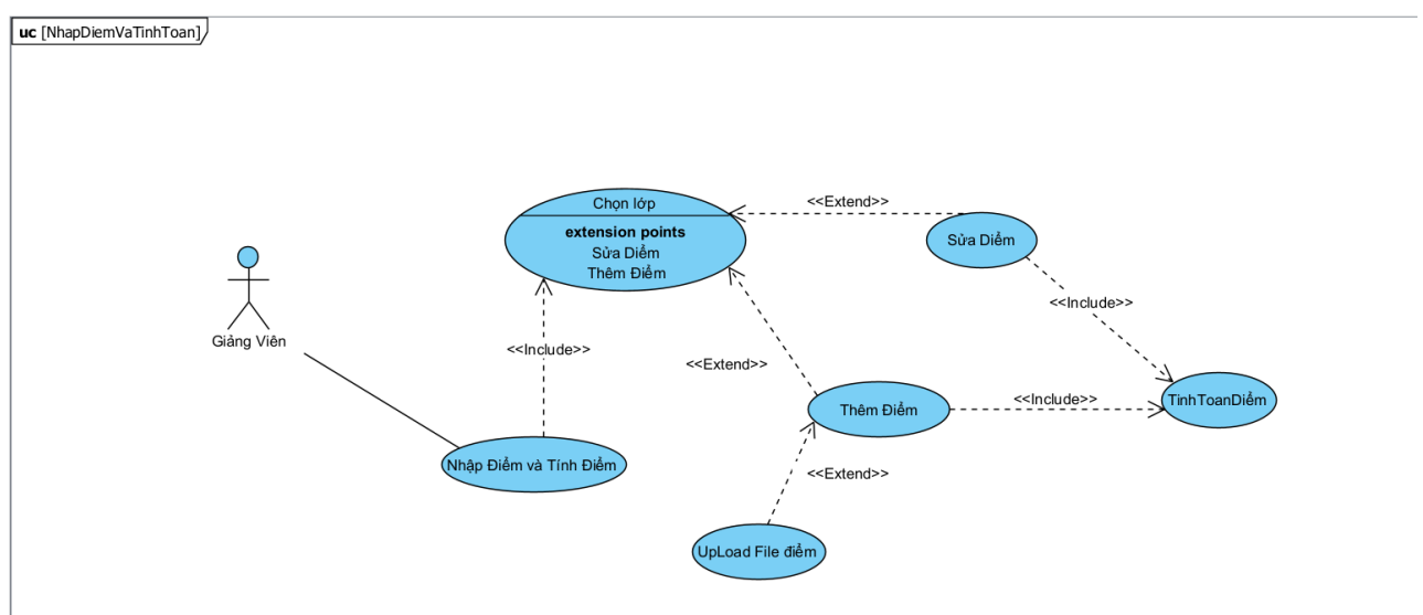
Hình 3. 8: Biểu đồ use-case NhapDiemVaTinhToan
