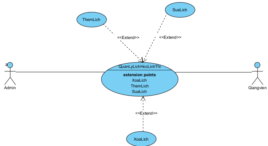
Hình 3. 4: Biểu đồ use-case QuanLyLichHocLichThi
