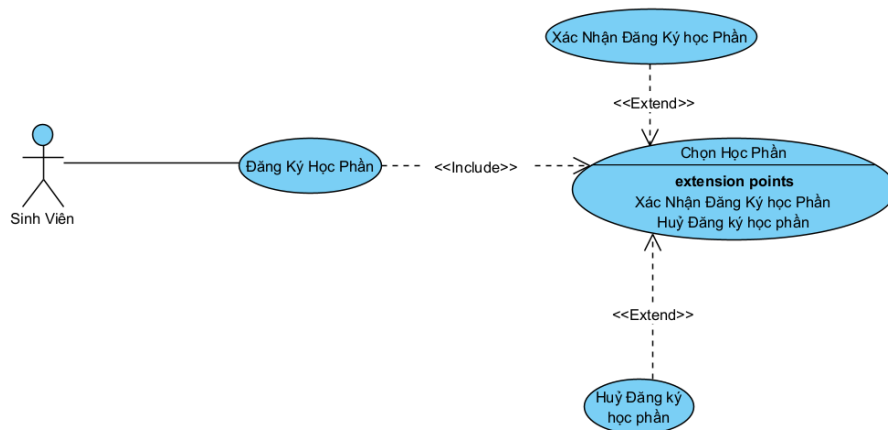
Hình 3. 10: Biểu đồ use-case DangKyHocPhan
