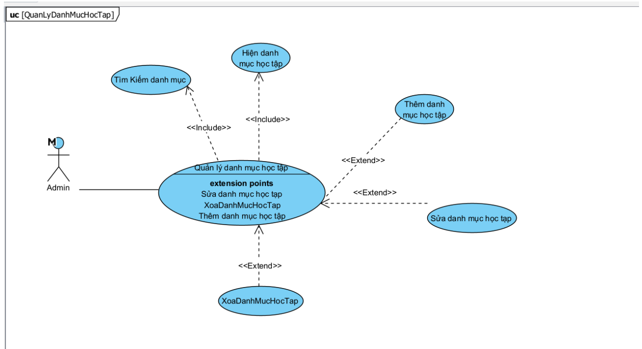
Hình 3. 2: Biểu đồ use-case QuanLyDanhMucHocTap
