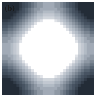
Voronoi
