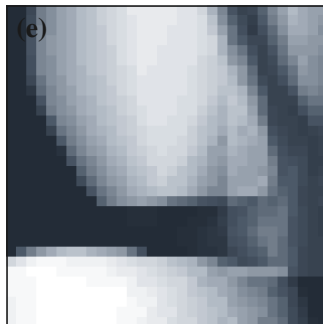
Voronoi
