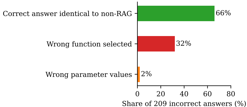
RAG failure breakdown (CD+Q+RAG, 7B, 209 incorrect)
