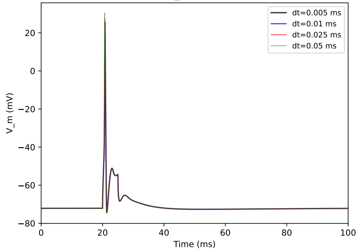
Somatic V_m for 4 dt values
