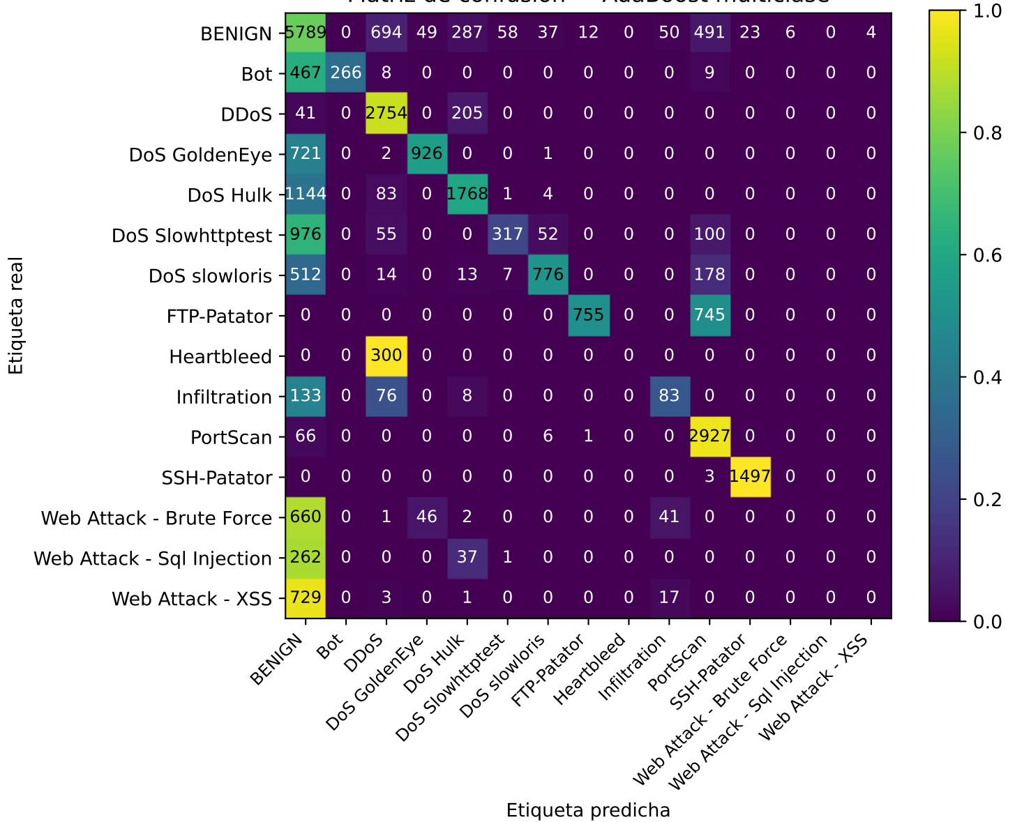
Matriz de confusión — AdaBoost multiclase
