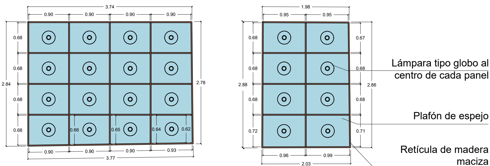
DET-01 PANELES DE ESPEJO
