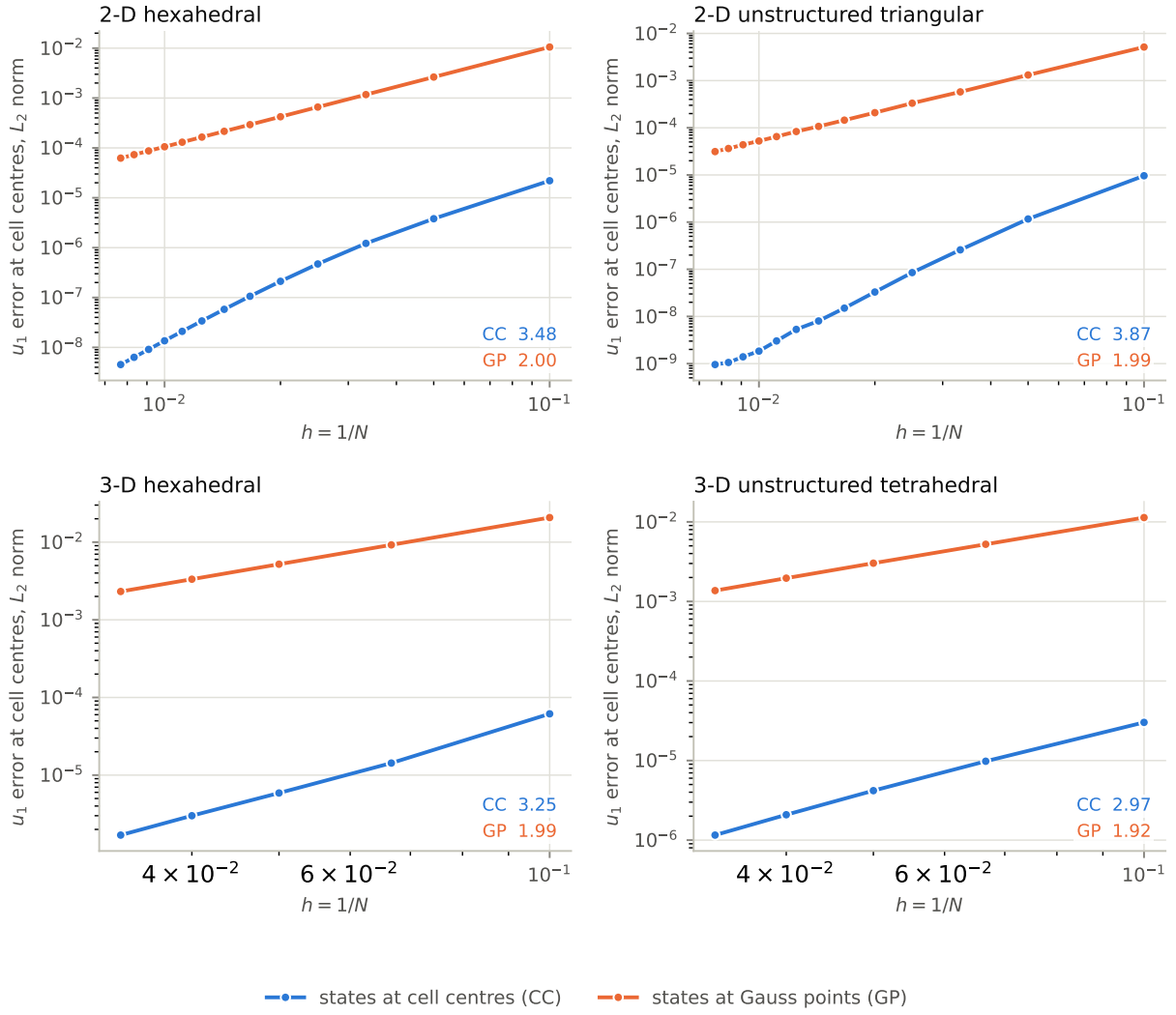
Figura 3: Error del estado iónico u_1 en centros de celda, cellCentredReconstruct contra gaussPointODE , con la tríada (p_3, \cdot, p_3) . El modo de puntos de Gauss queda clavado en orden dos en los cuatro paneles; el centrado en celda sigue al esquema. Generada por figures/fig_orders.py .
