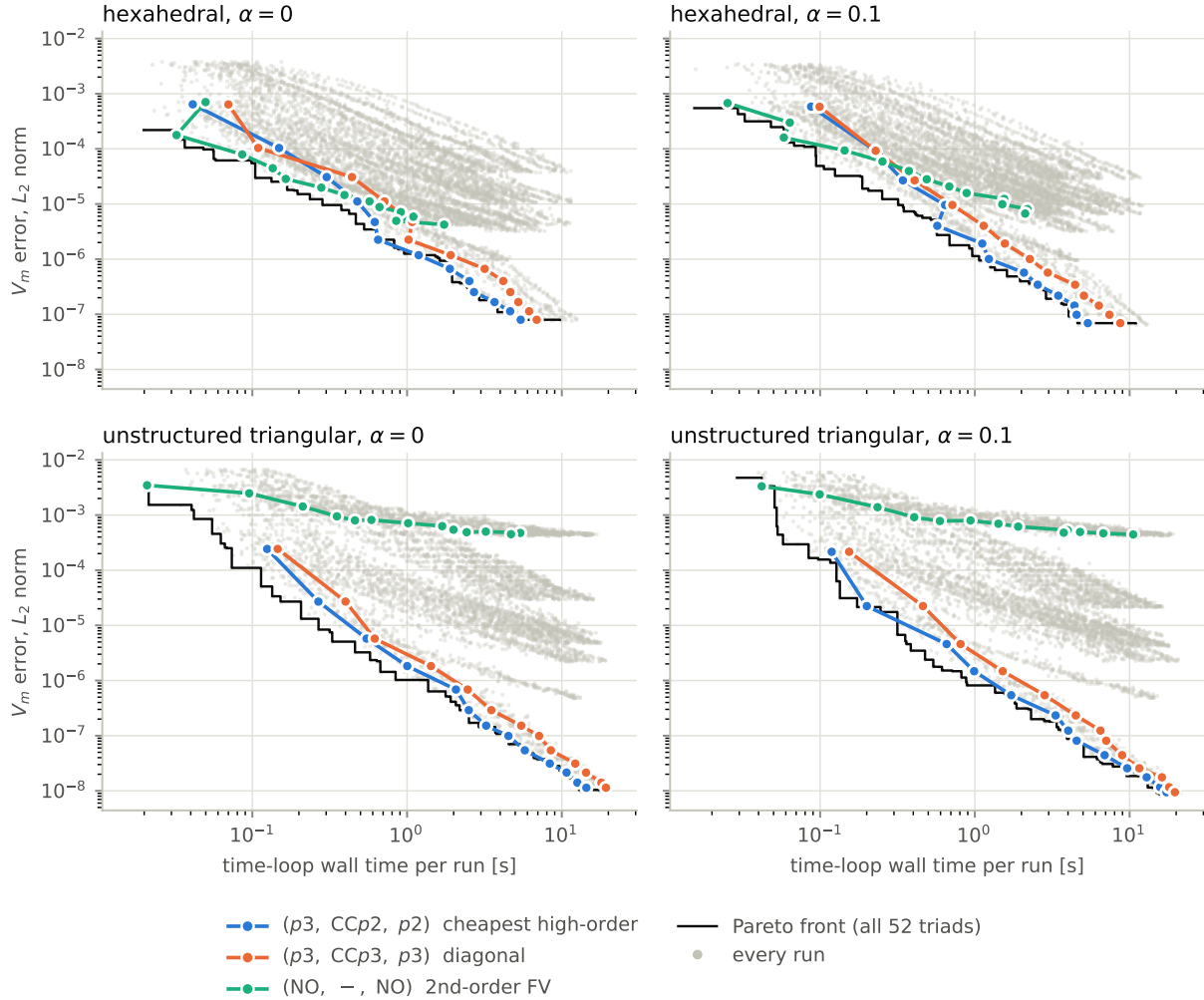
Figura 1: Frente de Pareto de precisión contra costo sobre el espacio de tríadas ( V_m , estados, I_{ion} ), del barrido con np=4 , Picard y \Delta t = 10^{-3} , N = 10\text{--}130 . Cada punto tenue es una corrida; la curva escalonada negra es el frente no dominado; las tres curvas de color son trayectorias de refinamiento de malla para la tríada de alto orden más barata (p3, CCp2, p2) , la diagonal (p3, CCp3, p3) y el FV de segundo orden. La tríada diagonal queda por encima del frente en los cuatro paneles. Generada por figures/fig_pareto_triads.py a partir de figures/pareto_2d_picard_dt1e-3.csv .
