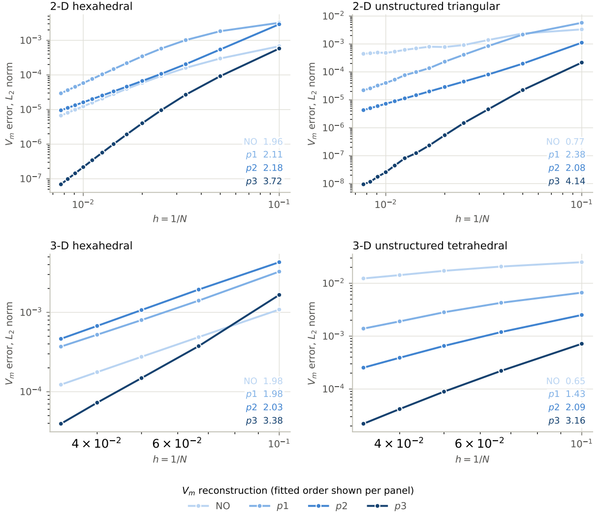
Figura 2: Orden espacial de V_m para los cuatro niveles de reconstrucción de la diagonal, en 2D ( N = 10 –130) y 3D ( N = 10 –30), sobre mallas estructuradas y no estructuradas. El número de cada panel es el orden ajustado sobre todo el rango de ese panel. Los cuatro niveles son una escala ordenada, así que se dibujan como un solo tono de claro a oscuro y no como cuatro colores categóricos. Generada por figures/fig.orders.py a partir de los archivos errors_vs_N crudos.
