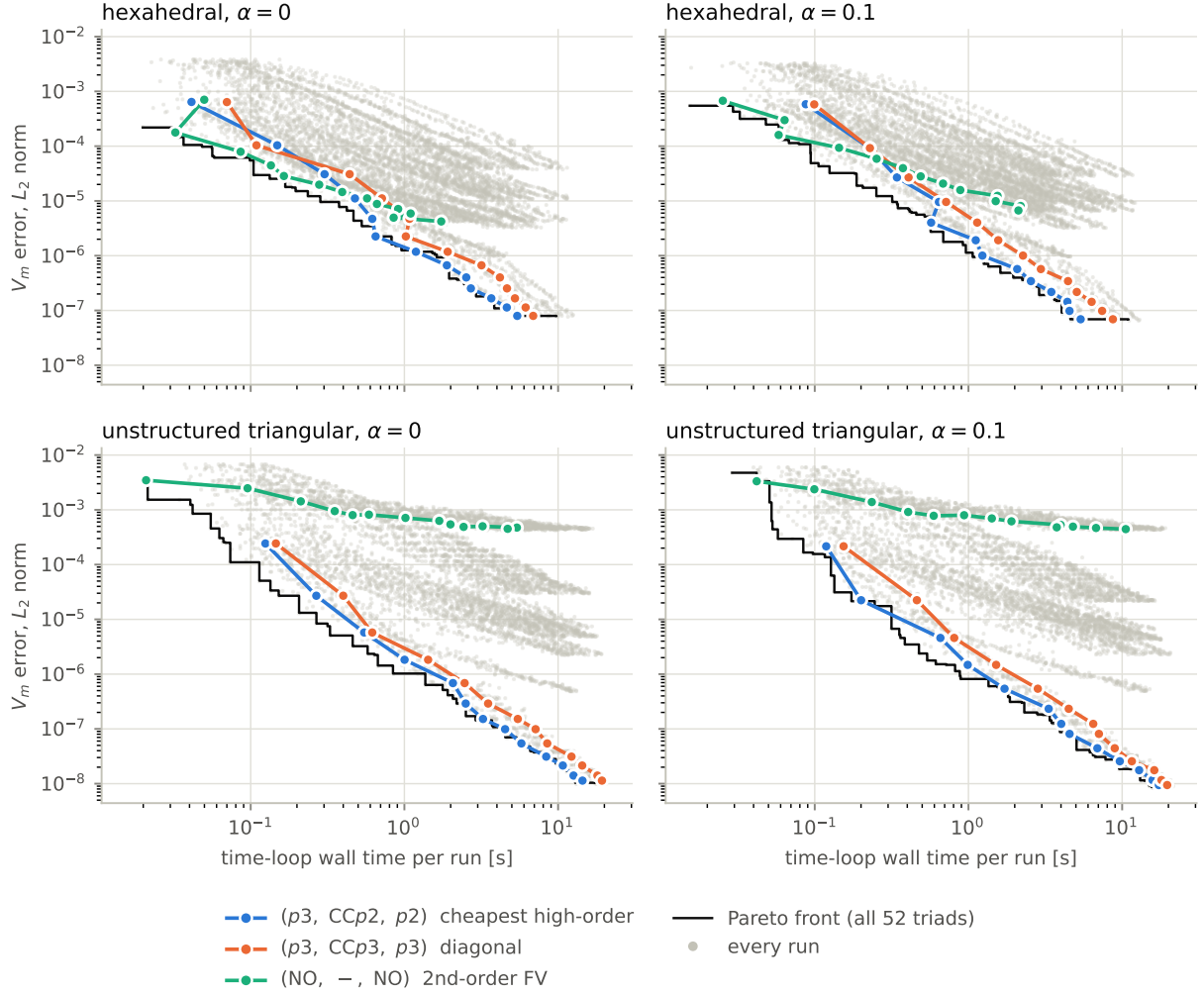
Figura 1: Frente de Pareto de precisión contra costo sobre el espacio de tríadas ( V_m , estados, I_{ion} ), del barrido con np=4 , Picard y \Delta t = 10^{-3} , N = 10-130 . Cada punto tenue es una corrida; la curva escalonada negra es el frente no dominado; las tres curvas de color son trayectorias de refinamiento de malla para la tríada de alto orden más barata ( p3, CCp2, p2 ), la diagonal ( p3, CCp3, p3 ) y el FV de segundo orden. La tríada diagonal queda por encima del frente en los cuatro paneles. Generada por figures/fig_pareto-triads.py a partir de figures/pareto_2d_picard_dt1e-3.csv .
