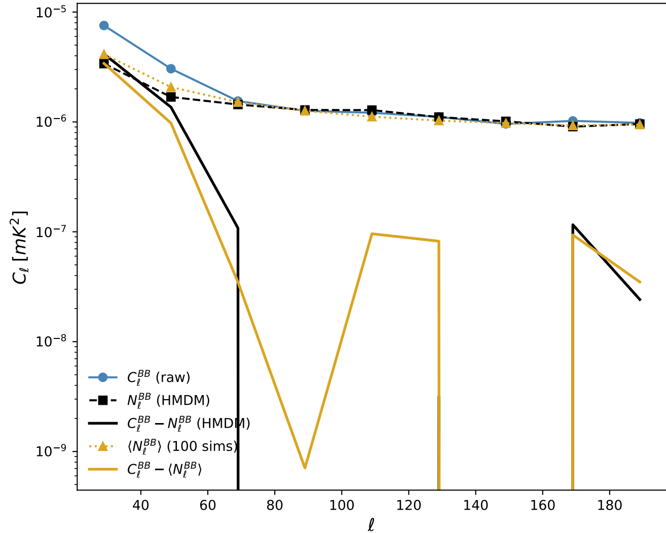
QUIJOTE 11 GHz — BB
