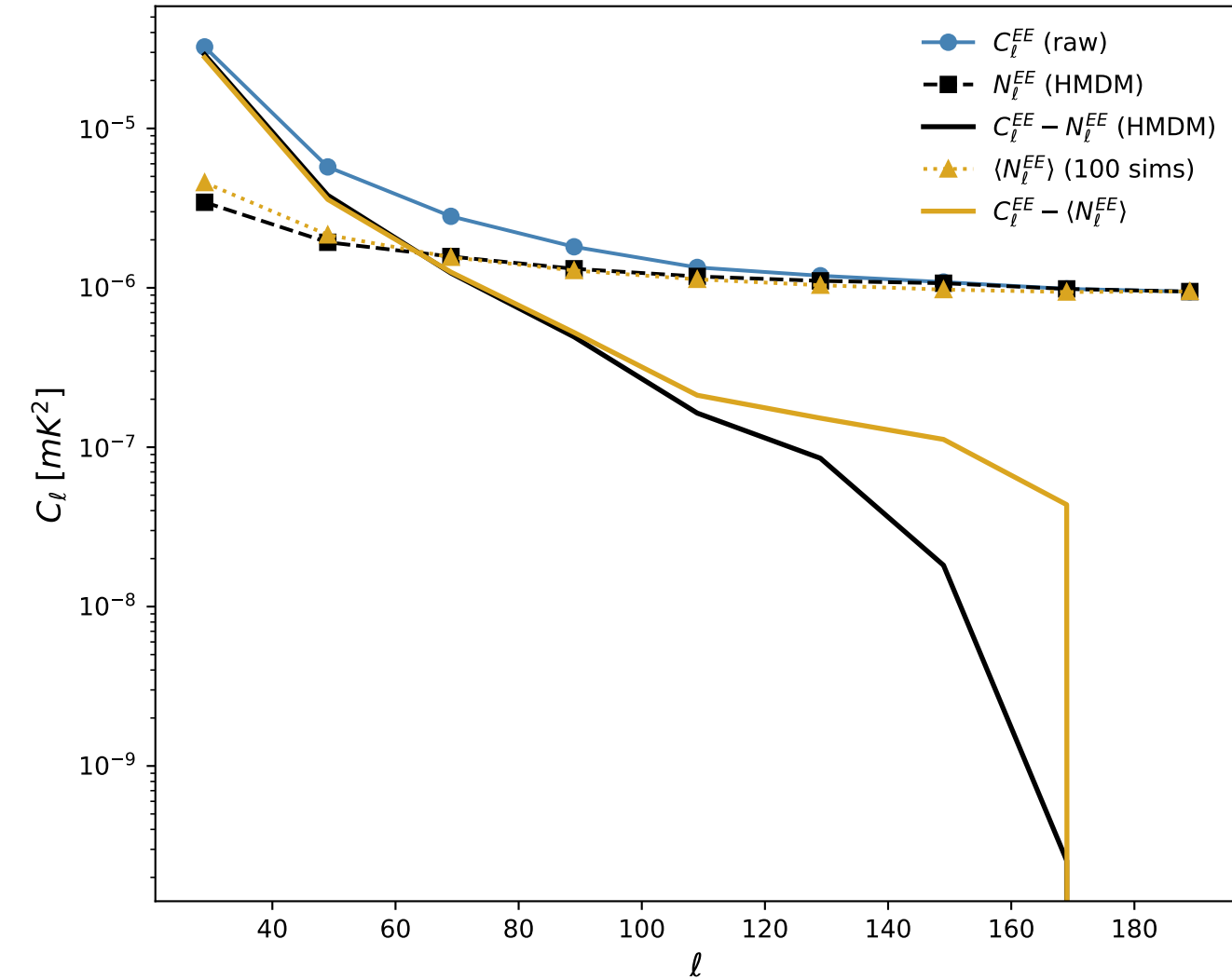
QUIJOTE 11 GHz — EE
