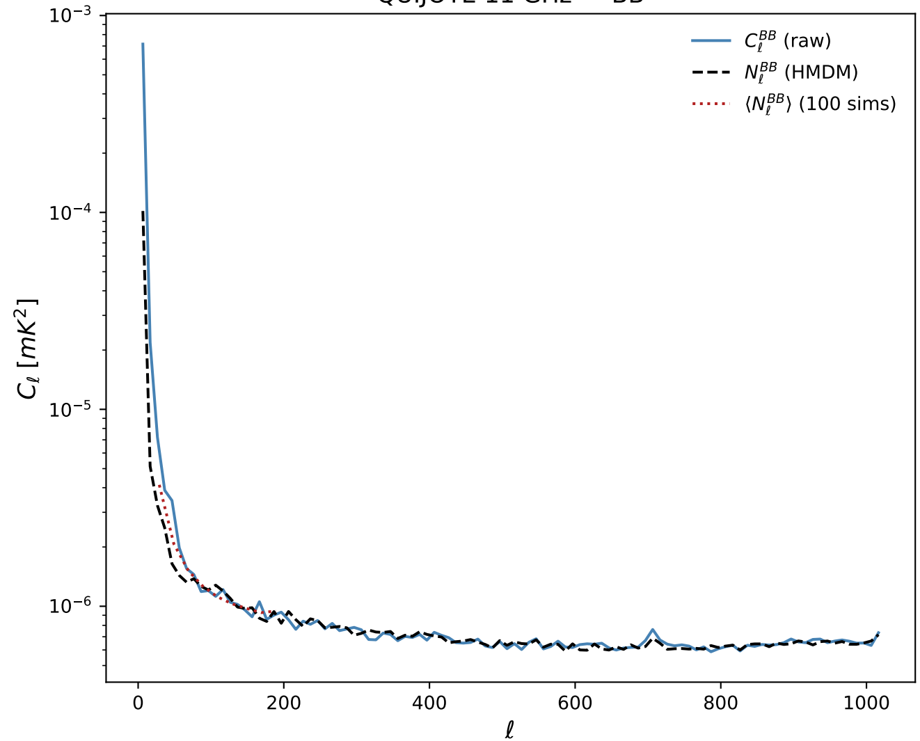
QUIJOTE 11 GHz — BB
