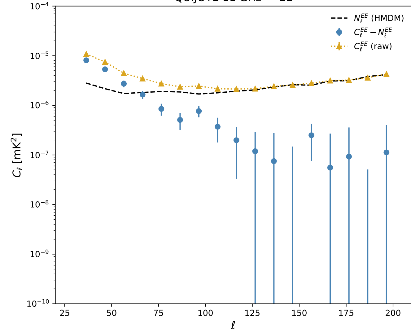
QUIJOTE 11 GHz — EE
