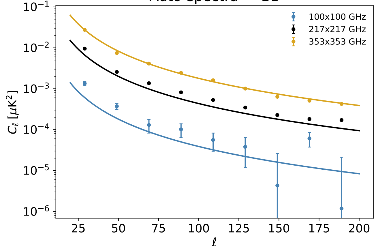
Auto-spectra — BB
