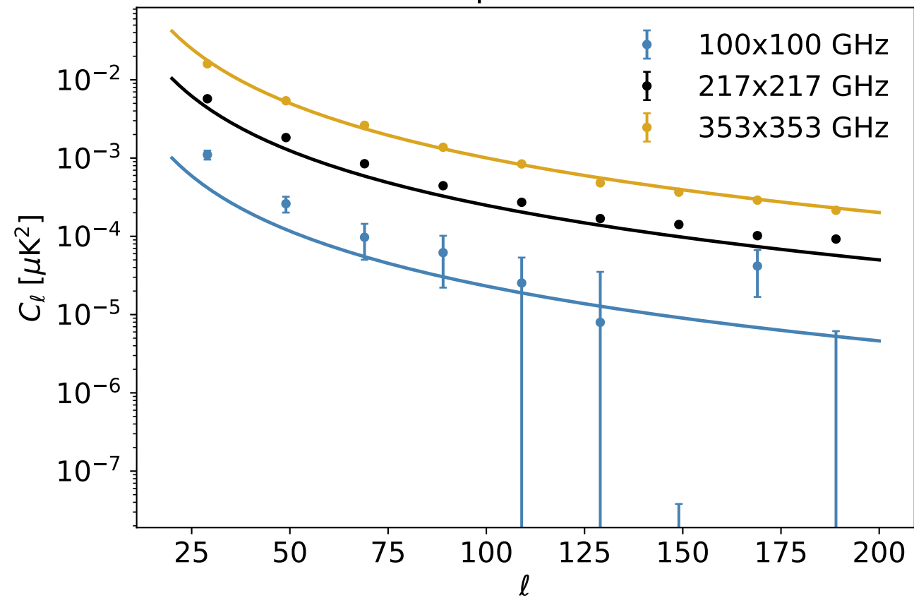
Auto-spectra — BB
