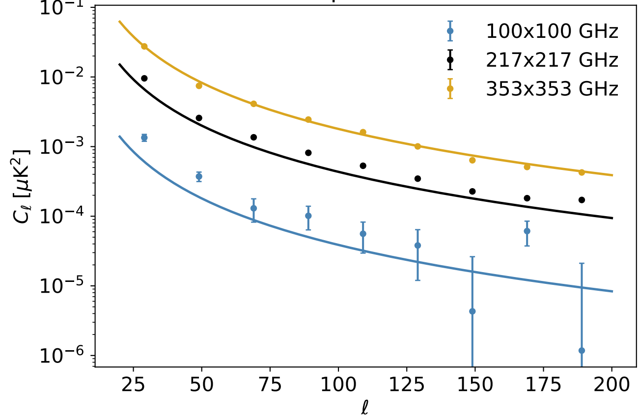
Auto-spectra — BB
