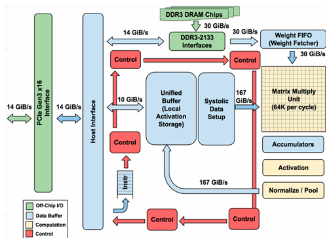
Figura 3: Diagrama de bloques de la TPU v1. El núcleo de cómputo es la Matrix Multiply Unit (amarillo). Sus entradas son el Weight FIFO y el Unified Buffer (azul), y su salida se deposita en los Accumulators . La unidad de activación aplica funciones no lineales sobre los acumuladores antes de devolver el resultado al Unified Buffer [7].
