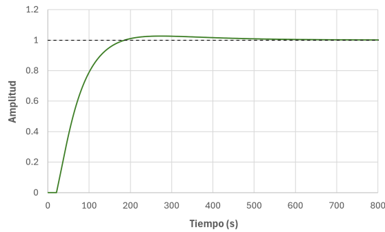
Fig III.1: Respuesta del sistema con controlador PI diseñado en CSD.
