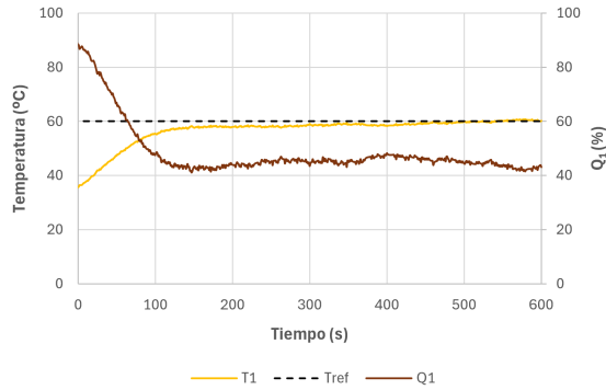
Fig VI.1: Evolución de la implementación experimental a T_{ref} = 60 °C
