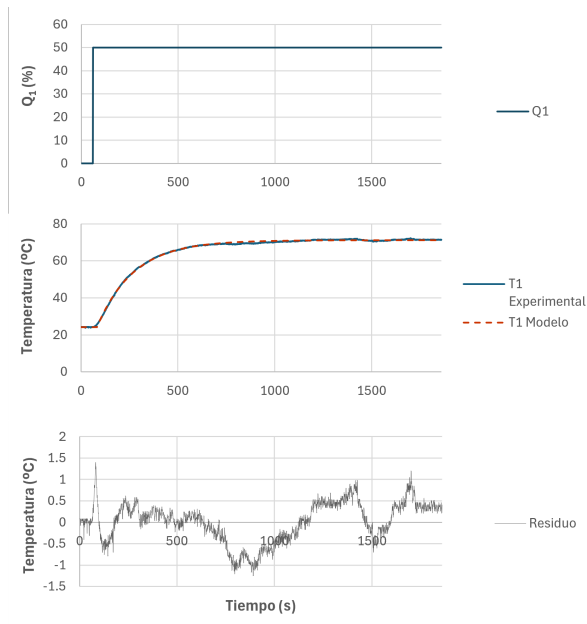
Fig V.1: Identificación FOPDT del ensayo escalón
