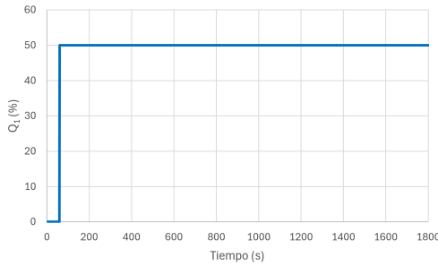
Fig VI.5: Entradas tipo escalón aplicadas al sistema
