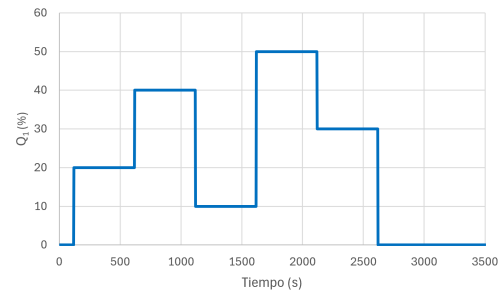
Fig VI.2: Entradas tipo escalón aplicadas al sistema
