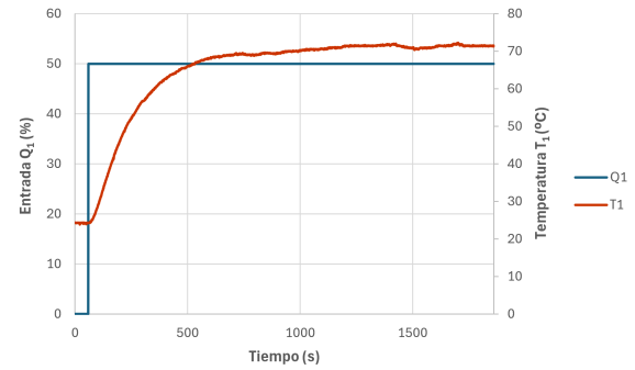
Fig IV.1: Ensayo escalón aplicado al sistema, con Q_1 fijado en 50 %
