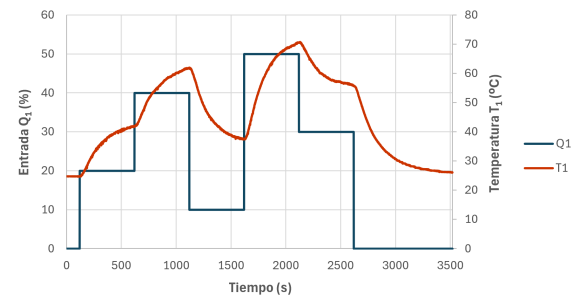
Fig IV.2: Ensayo multinivel aplicado al sistema
