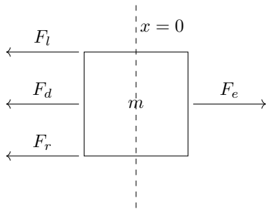
Fig III.1: Diagrama de cuerpo libre del solenoide.
