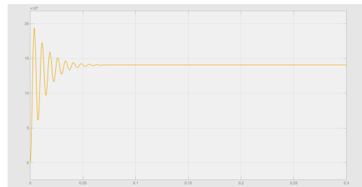
Fig VII.4: Respuesta al escalón del sistema completo en Simscape (presión con respecto al tiempo)
