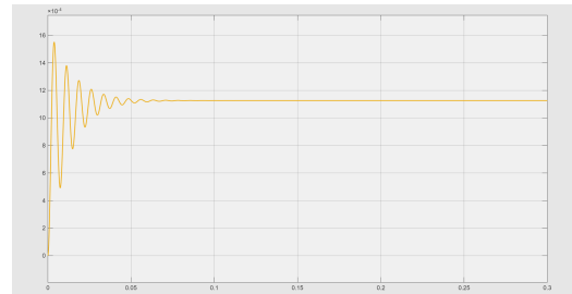
Fig VII.3: Desplazamiento del émbolo en Simscape (desplazamiento con respecto al tiempo)
