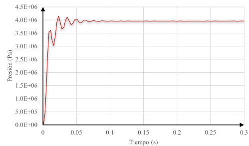
Fig VII.2: Respuesta al escalón de la TF
