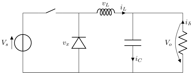
Fig II.1: Circuito equivalente del convertidor buck [1].
