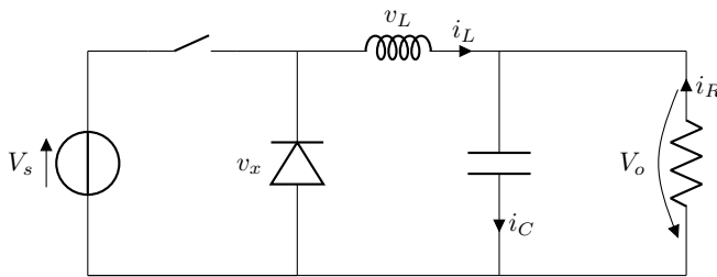
Fig II.1: Circuito equivalente del convertidor buck [hart2011].
