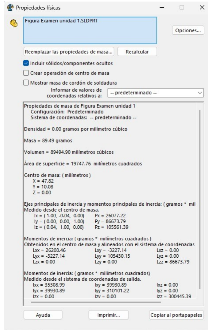
Figura 5. Propiedades de masa en SOLIDWORKS (volumen = 89 494.90 mm 3 )
