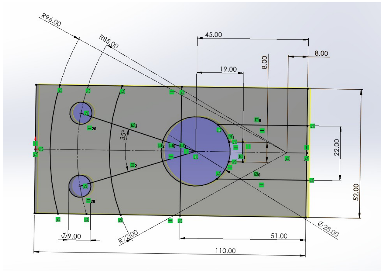
Figura 6. Croquis con cotas y relaciones
