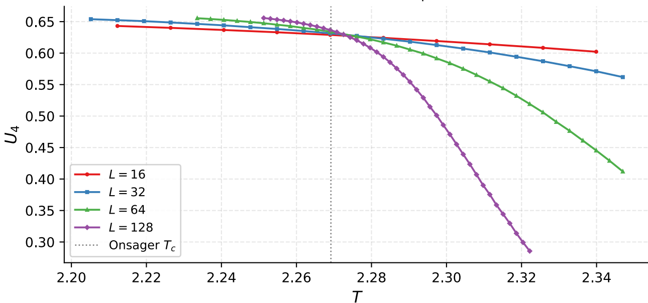
Cumulante de Binder U_4 — Wolff
