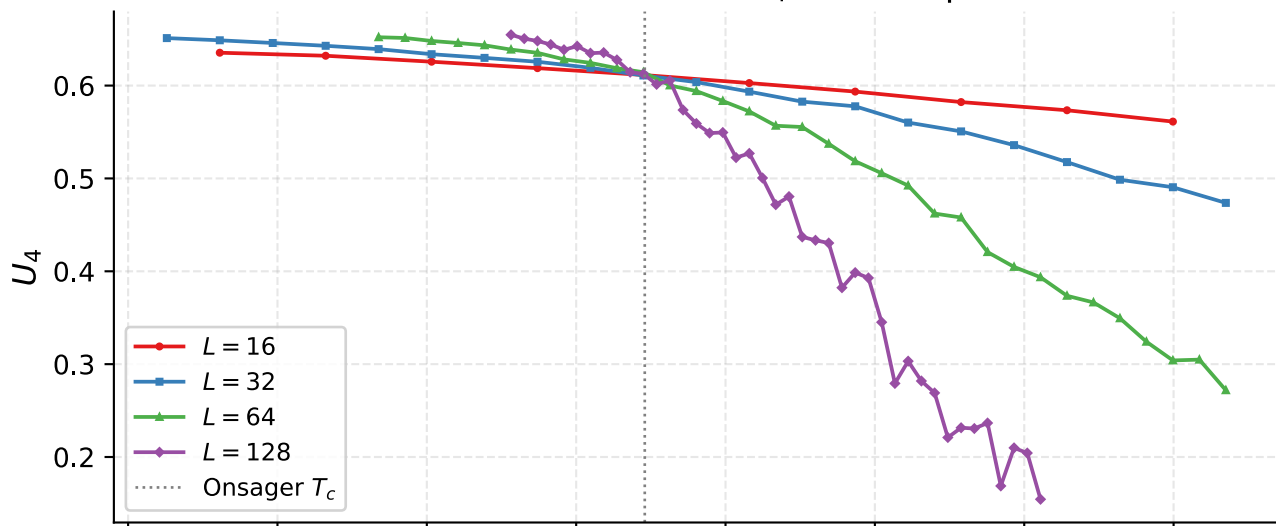
Cumulante de Binder U_4 — Metropolis
