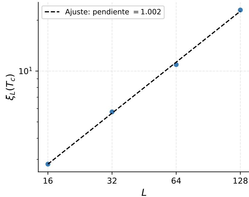
\xi_L(T_c) vs L — Metropolis
