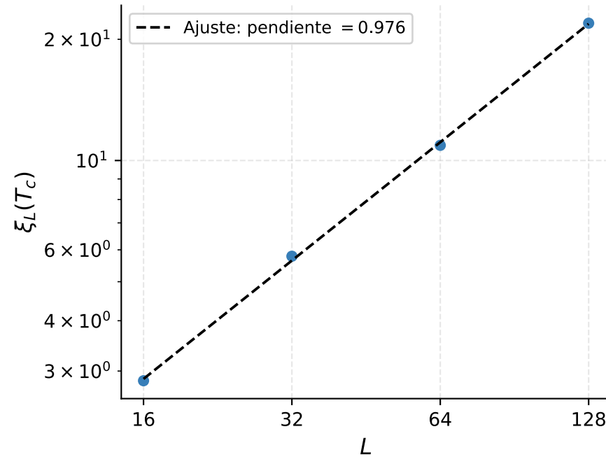
\xi_L(T_c) vs L — Glauber
