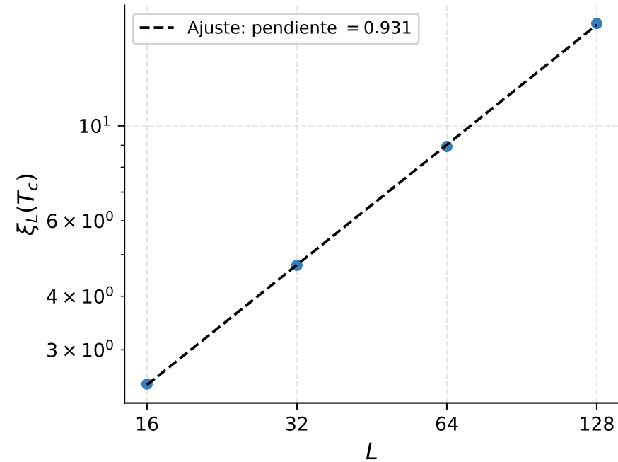
\xi_L(T_c) vs L — Wolff
