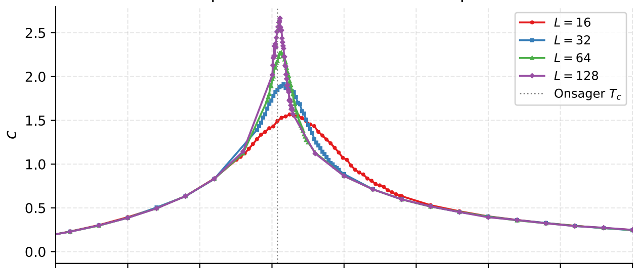
Capacidad calorífica c — Glauber
