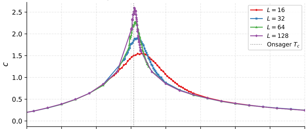
Capacidad calorífica c — Wolff
