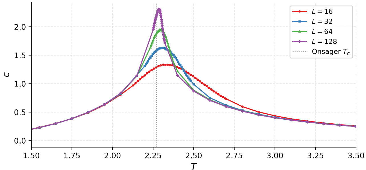
Capacidad calorífica c — Wolff
