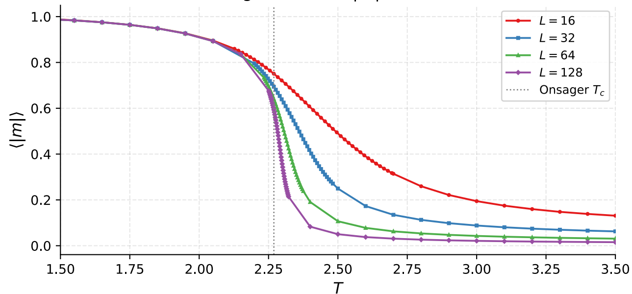
Magnetización \langle |m| \rangle — Wolff
