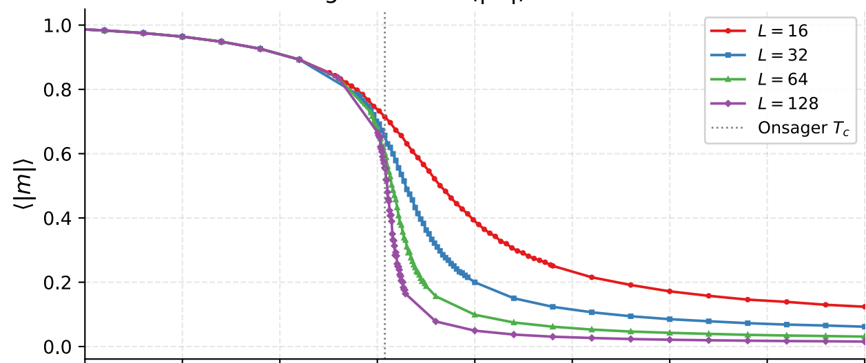
Magnetización \langle |m| \rangle — Glauber
