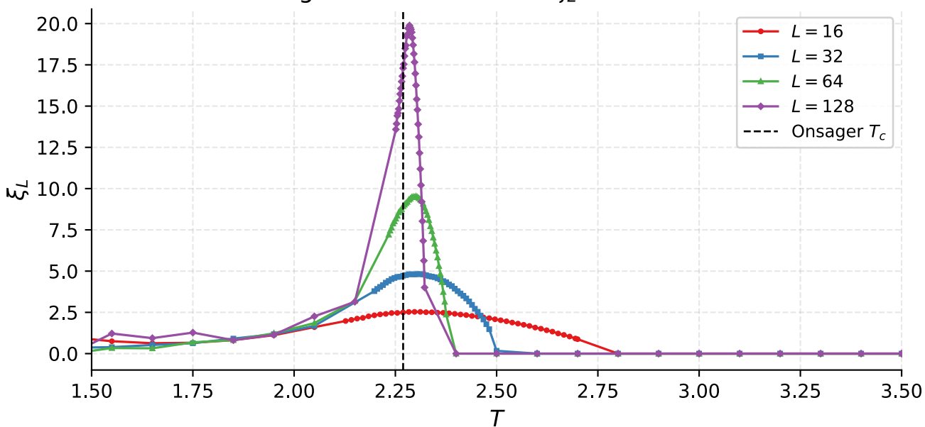
Longitud de correlación \xi_L vs T — Wolff
