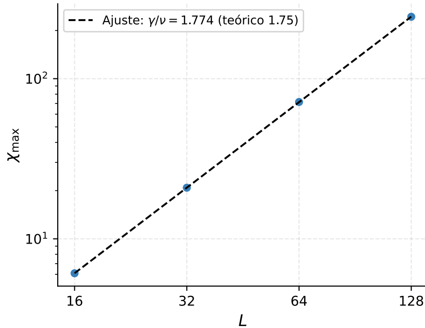
\chi_{\max} vs L — Glauber
