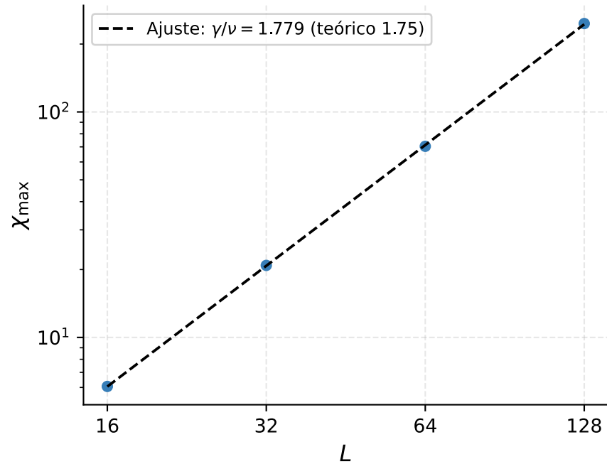
\chi_{\max} vs L — Metropolis
