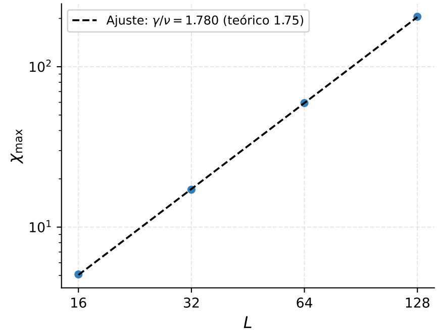
\chi_{\max} vs L — Wolff
