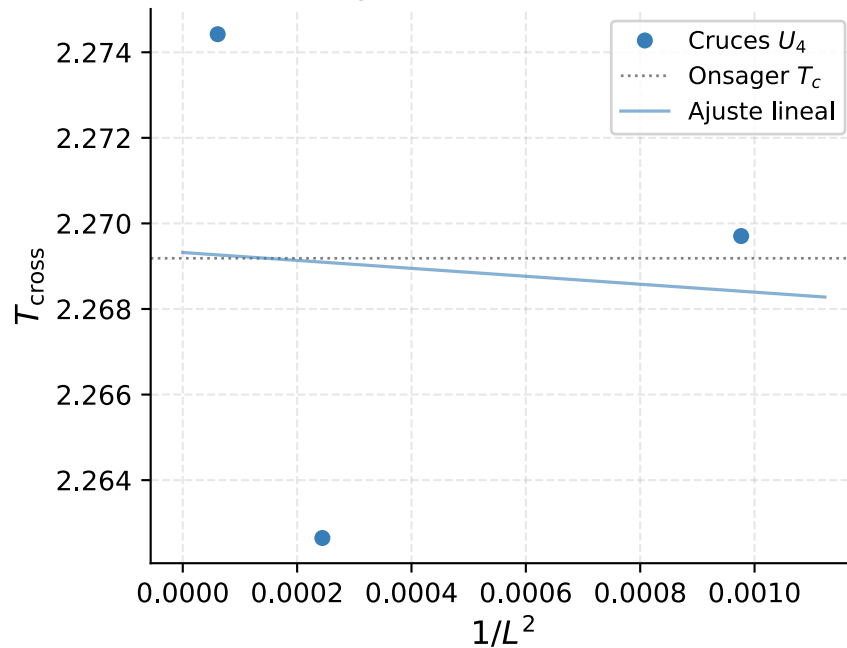
Extrapolación T_c — Glauber
