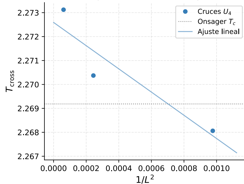
Extrapolación T_c — Metropolis
