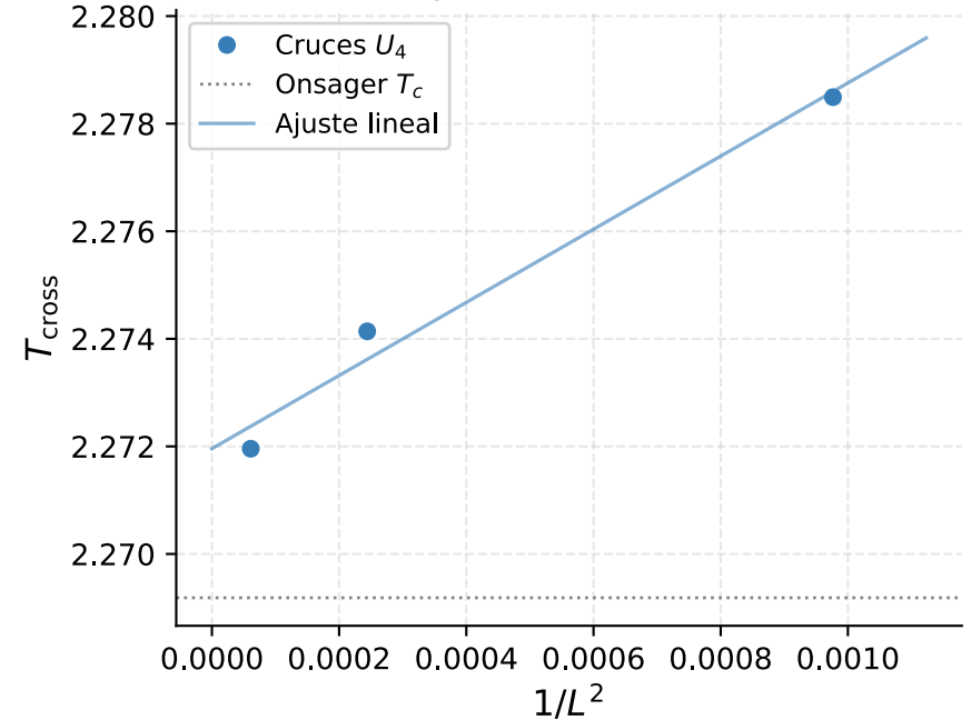
Extrapolación T_c — Wolff
