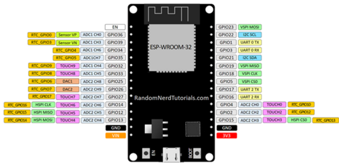
Figura 1: Pinout del ESP 32- 30 pines
