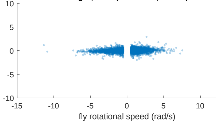
dLight, dark (n=198881, r=0.16)
