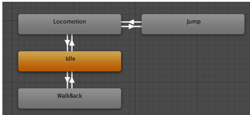
Figura 2.3: Captura del sistema de animaciones de Unity, estructurado en forma de una HFSM en la que los nodos naranja son “superestados”. Fuente: https://docs.unity3d.com/560/Documentation/Manual/StateMachineBasics.html
