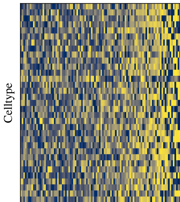
sctransform v2
