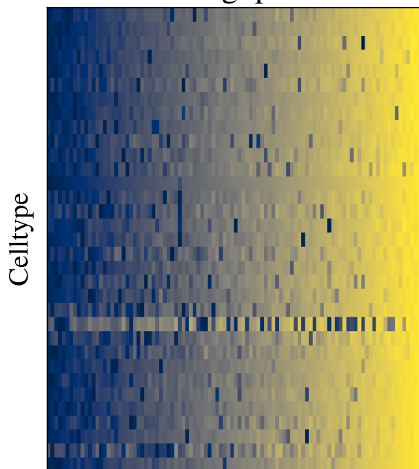
PFlog1pPF
