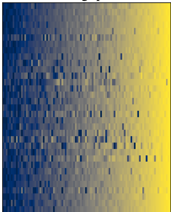
PFlog1pPF
