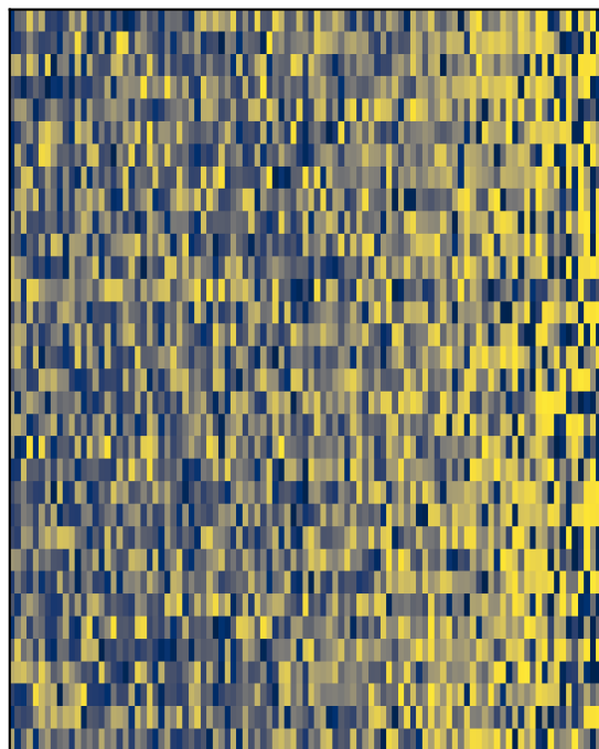
sctransform v2
