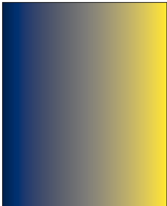
raw
