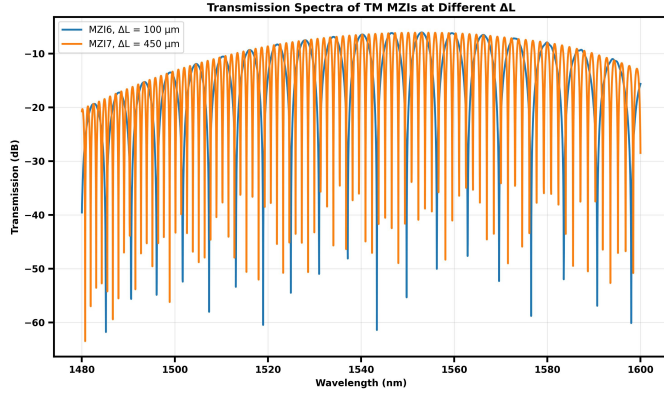
Fig. 15. Spectra of TM MZIs
