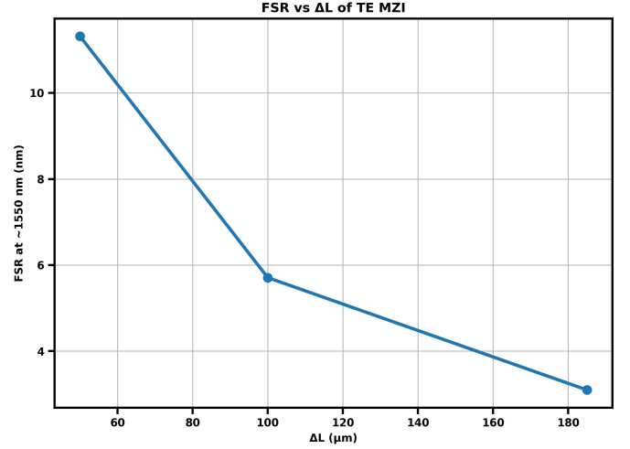
Fig. 12. FSR values vs \Delta L
