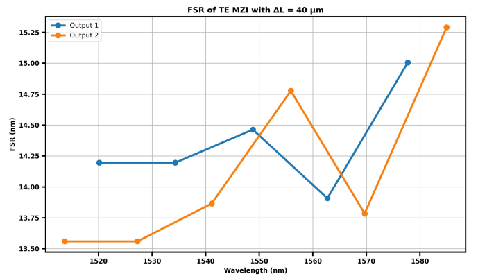
Fig. 14. FSR of TE MZI2
